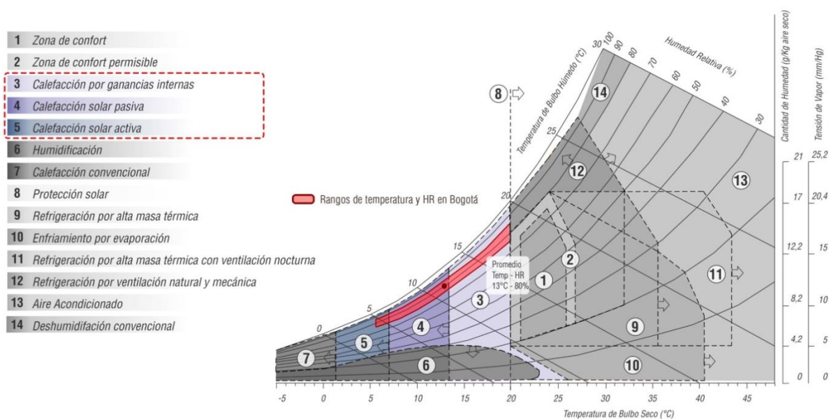
Figura 44. Diagrama de Givoni para Bogotá D.C.
