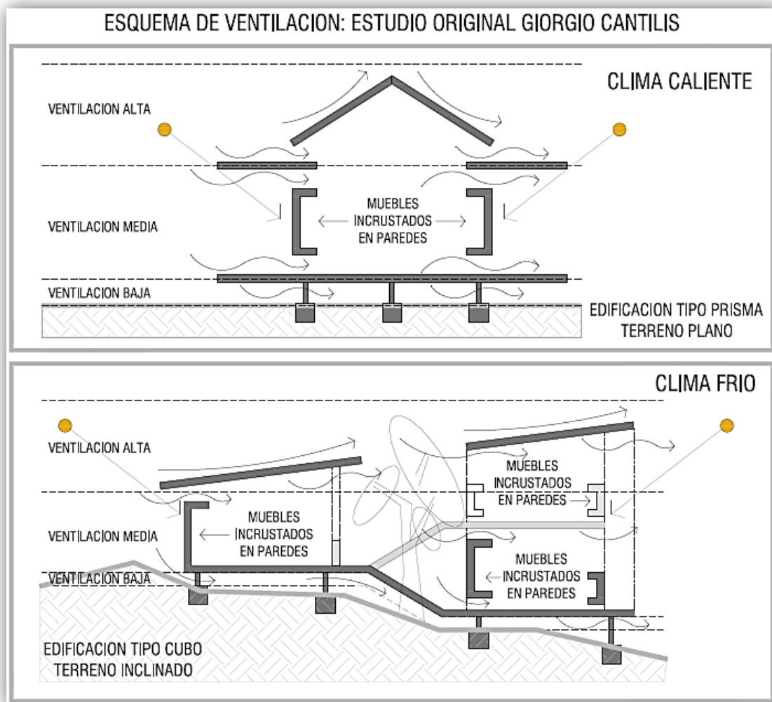
Figura 7. Esquema de ventilación: Estudio original Giorgio Cantili
