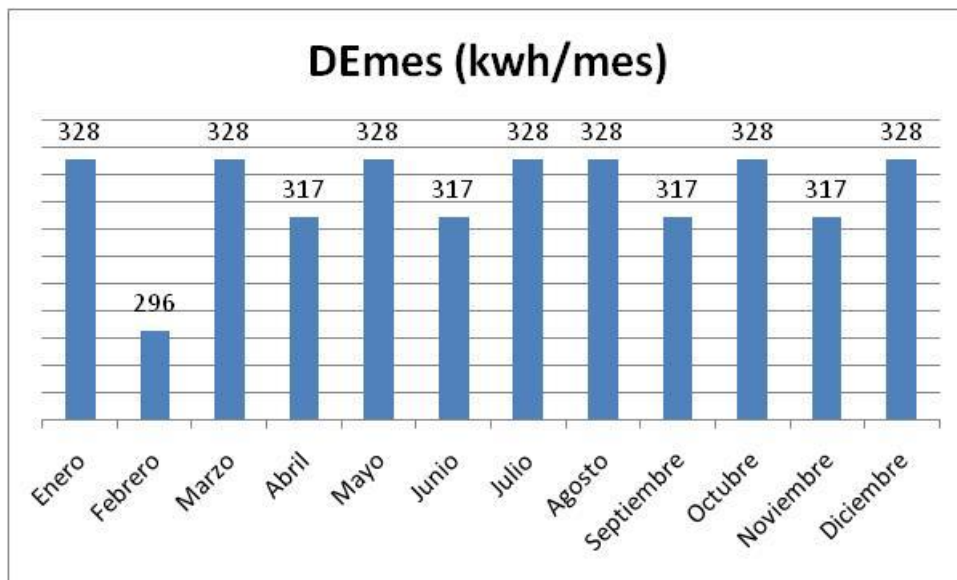
Gráfico 66. Demanda mensual de ACS (elaboración propia)
