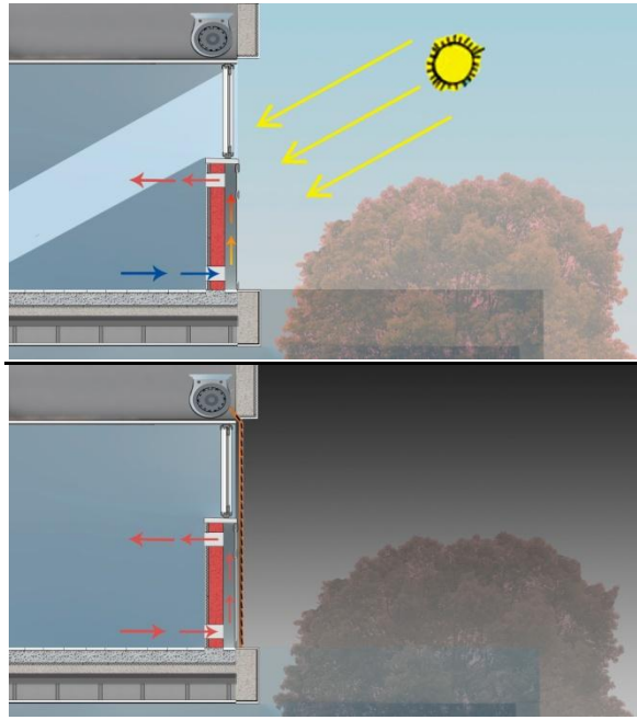
Imagen 14. Funcionamiento del Muro captador de calor en INVIERNO (día/noche)
