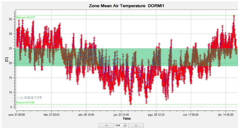
Gráfico 20. Temperatura Media anual. DORMITORIO1
