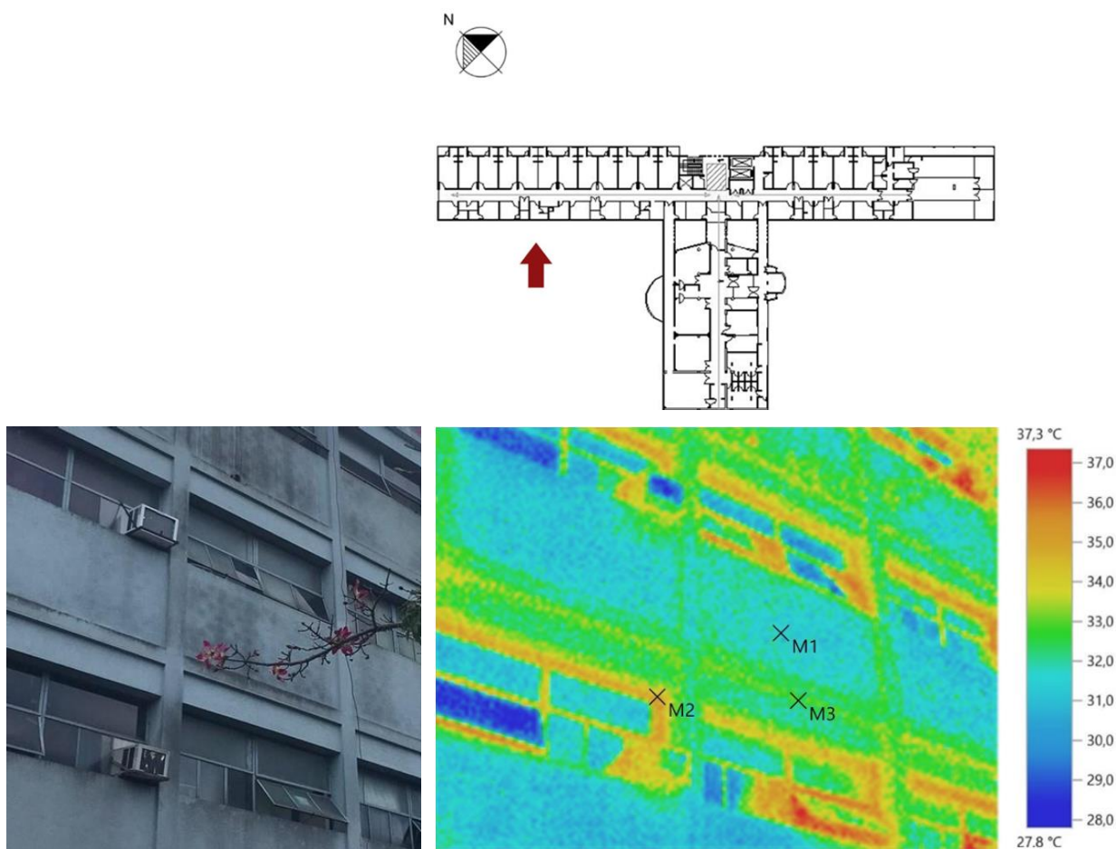
Figura 15: Imagen termográfica del área de internación del HIGA "San Roque" (orientación sur). Fuente: Elaboración propia
