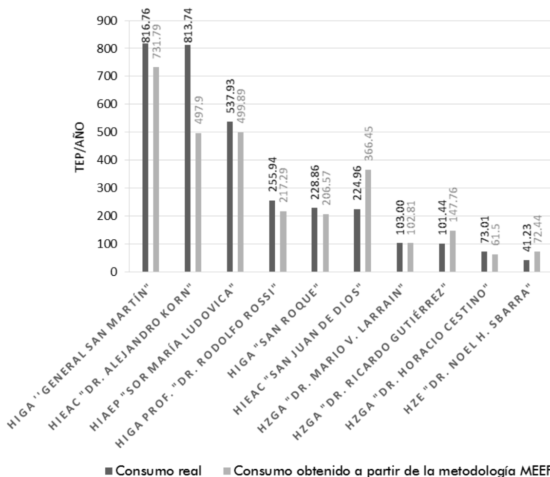
Gráfico 2: Consumos reales vs. Consumos obtenidos a partir de la aplicación de la metodología MEEP. Fuente: Elaboración propia
