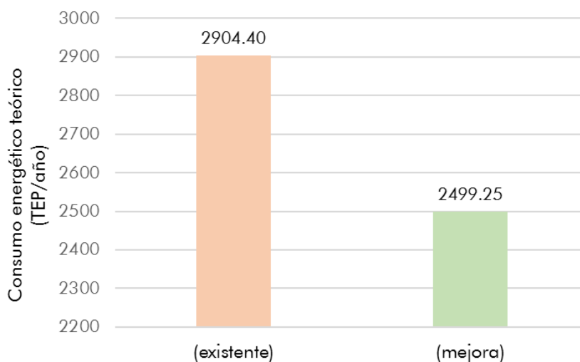
Gráfico 13: Estimación de la reducción teórica del consumo energético total de la red de salud en estudio. Fuente: Elaboración propia
