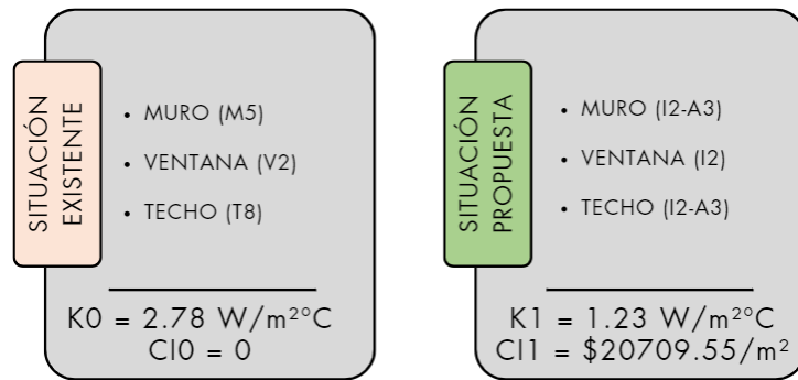
Figura 21: Síntesis de los valores de las variables K y CI correspondientes al área hospitalaria de internación.
