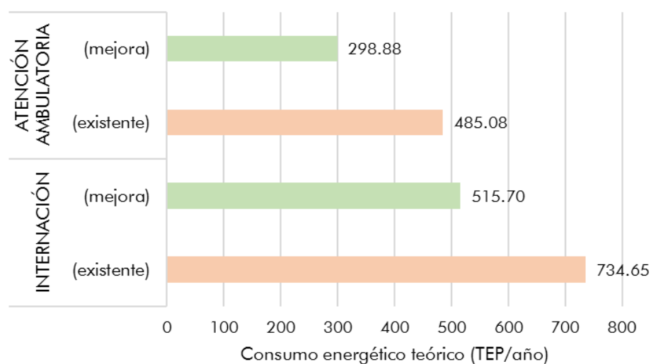
Gráfico 12: Estimación de la reducción teórica del consumo energético de las áreas de internación y atención ambulatoria de la red de salud en estudio. Fuente: Elaboración propia
