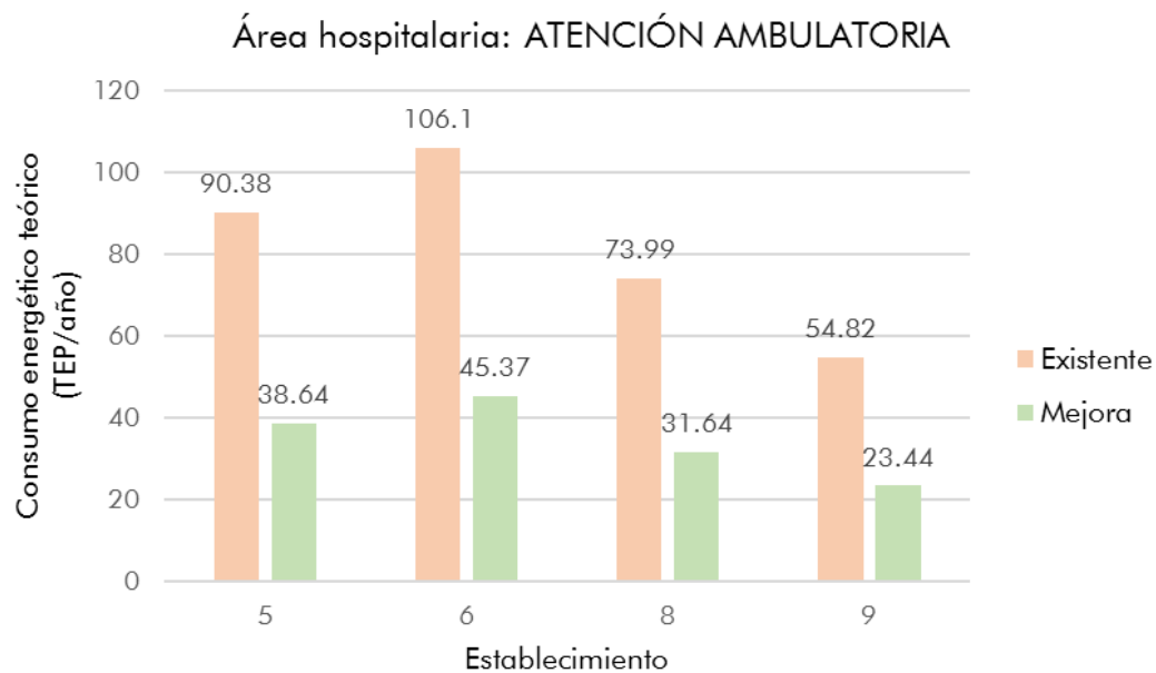
Gráfico 11: Estimación de la reducción del consumo energético a partir del reciclado de la envolvente edilicia del área de atención ambulatoria.
