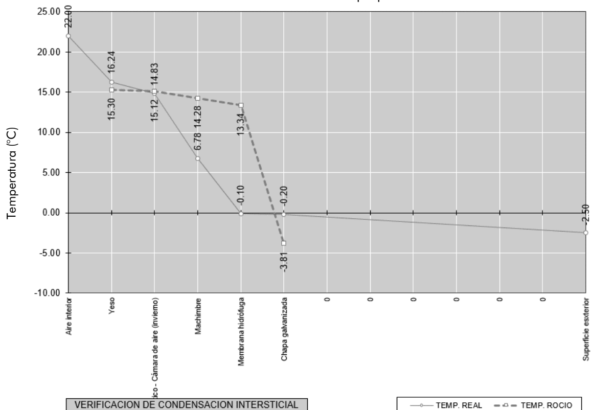
Gráfico 15: Verificación gráfica de condensación intersticial en la hoja "verifica" de la planilla CEEMACON.xls.
