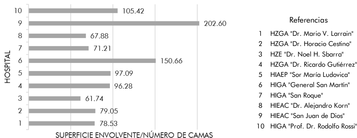
Gráfico 9: Valores del índice que relaciona la superficie de la envolvente con el número de camas, para cada hospital.
