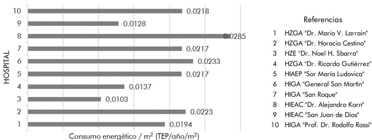
Gráfico 6: Relación entre el consumo energético real anual y la superficie de cada hospital. Fuente: Elaboración propia
