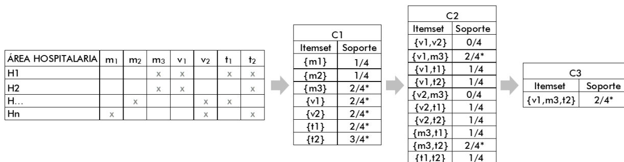
Figura 10: Procedimiento utilizado en el método de reglas de asociación para identificar elementos más frecuentes
