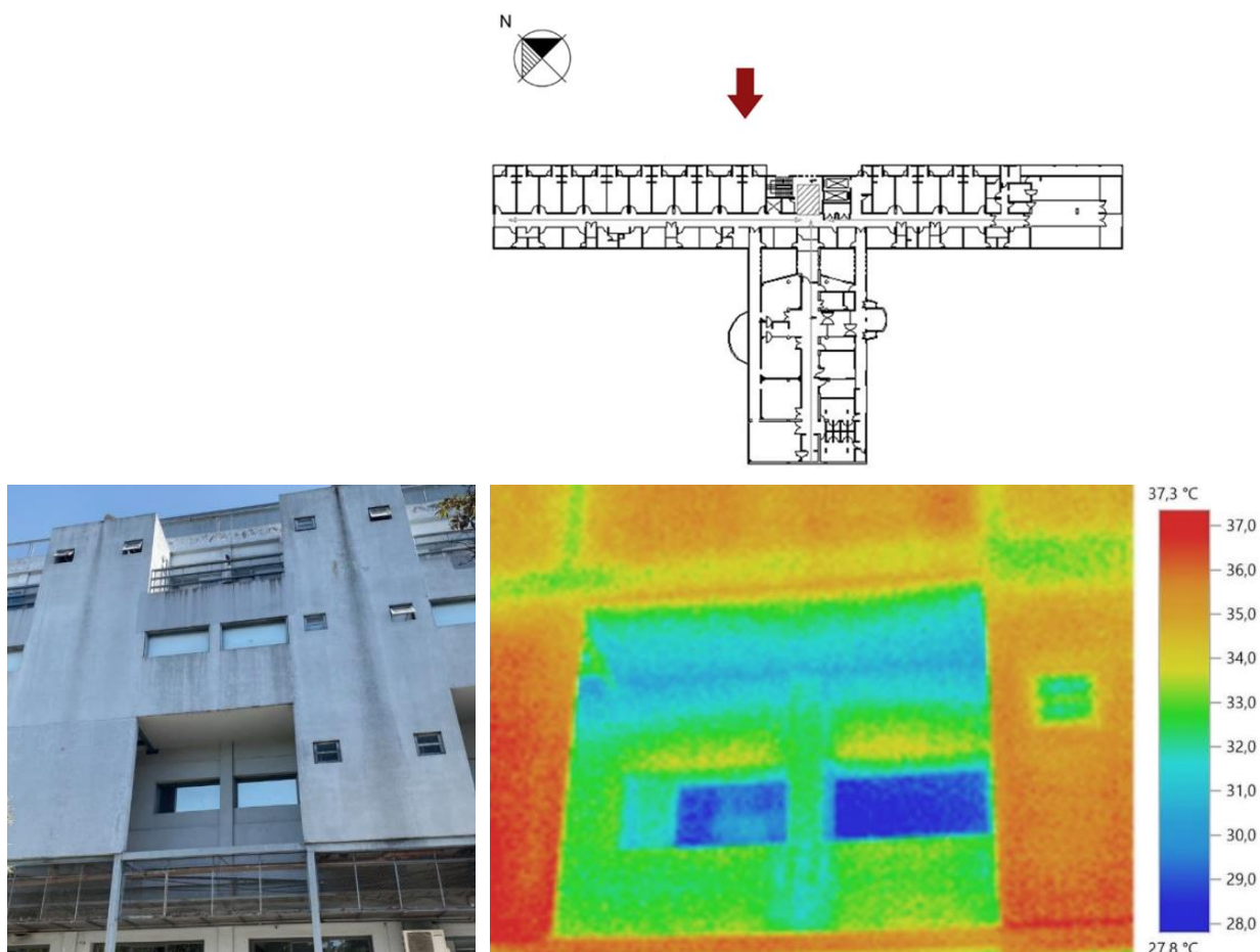
Figura 14: Imagen termográfica del área de internación del HIGA "San Roque" (orientación norte). Fuente: Elaboración propia
