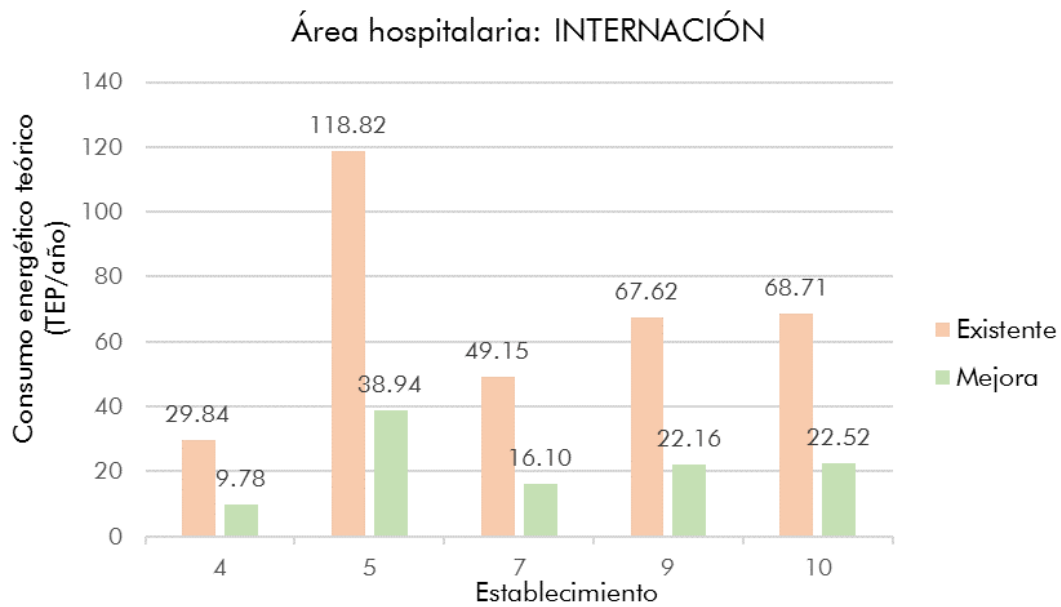
Gráfico 10: Estimación de la reducción del consumo energético a partir del reciclado de la envolvente edilicia del área de internación.
