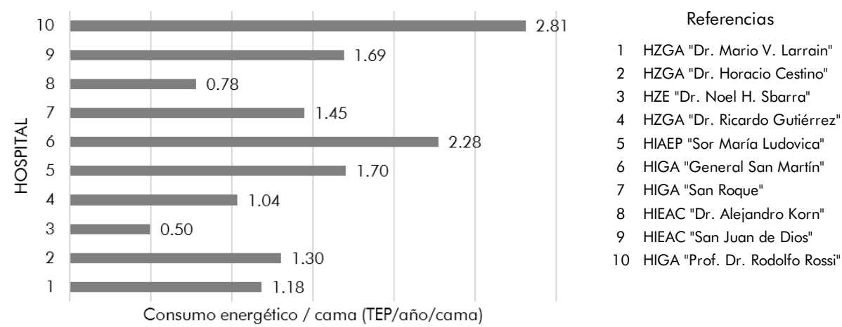
Gráfico 5: Relación entre el consumo energético real anual y la cantidad de camas de cada hospital. Fuente: Elaboración propia
