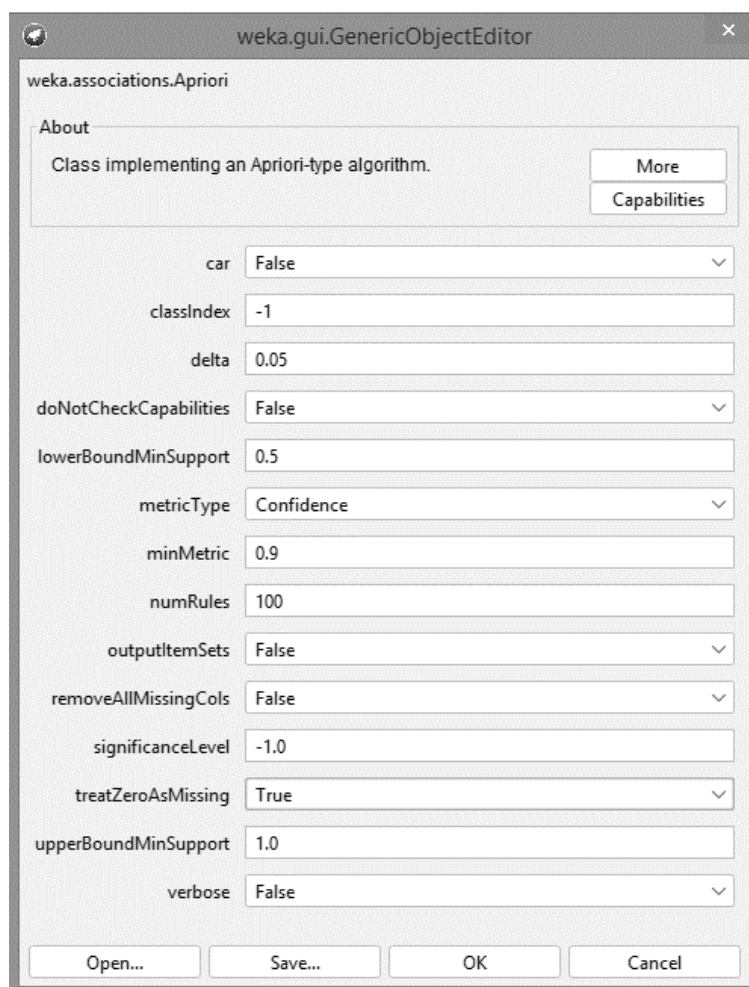
Figura 9: Configuración de parámetros en el software Weka. Fuente: Software WEKA.
