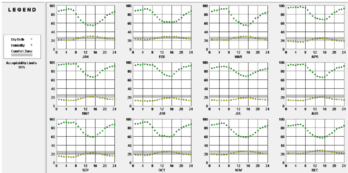
Figura 50: Humedad relativa mensual. Fuente: Climat Consultant.
