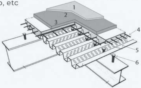
01.Terminación piso 02.Carpeta de nivelación 03.Contrapiso alivianado 04.Malla electrosoldada 05.Losa Steel deck: Capa de compresión y placa colaborante 06. Conector cortante
