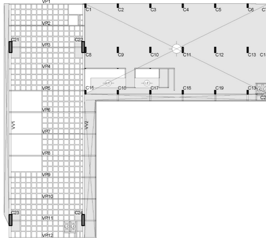
ESTRUCTURA PLANTA BAJA + 1.8m - Esc 1:500
