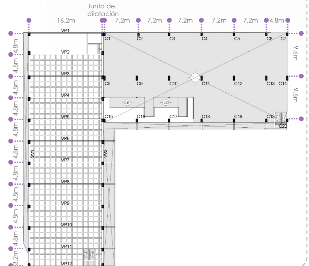
ESTRUCTURA PLANTA + 14,40m - Esc 1:500
