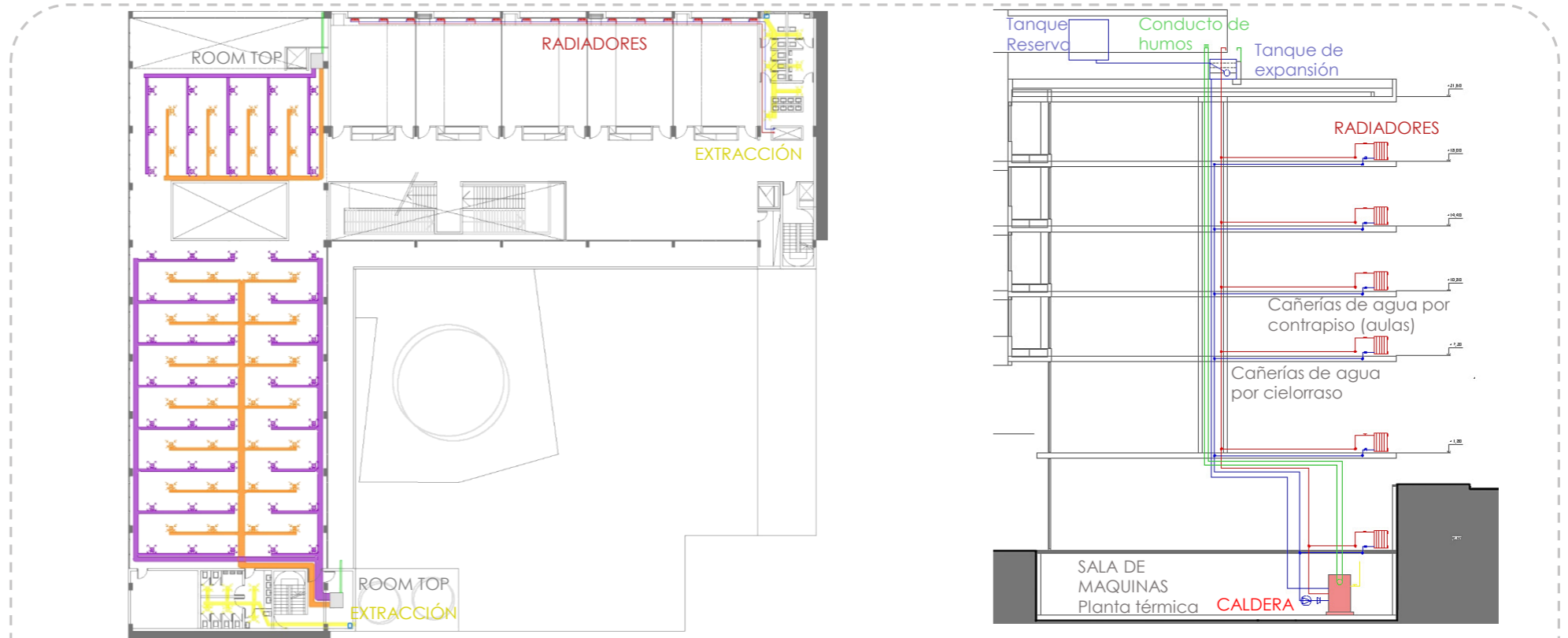
PLANTA +14.40 - Esc 1:500
