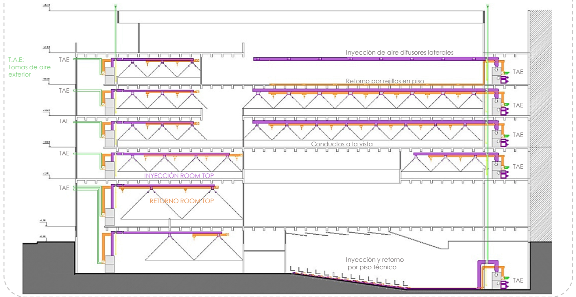
CORTE ACONDICIONAMIENTO DE AIRE - Esc 1:250
