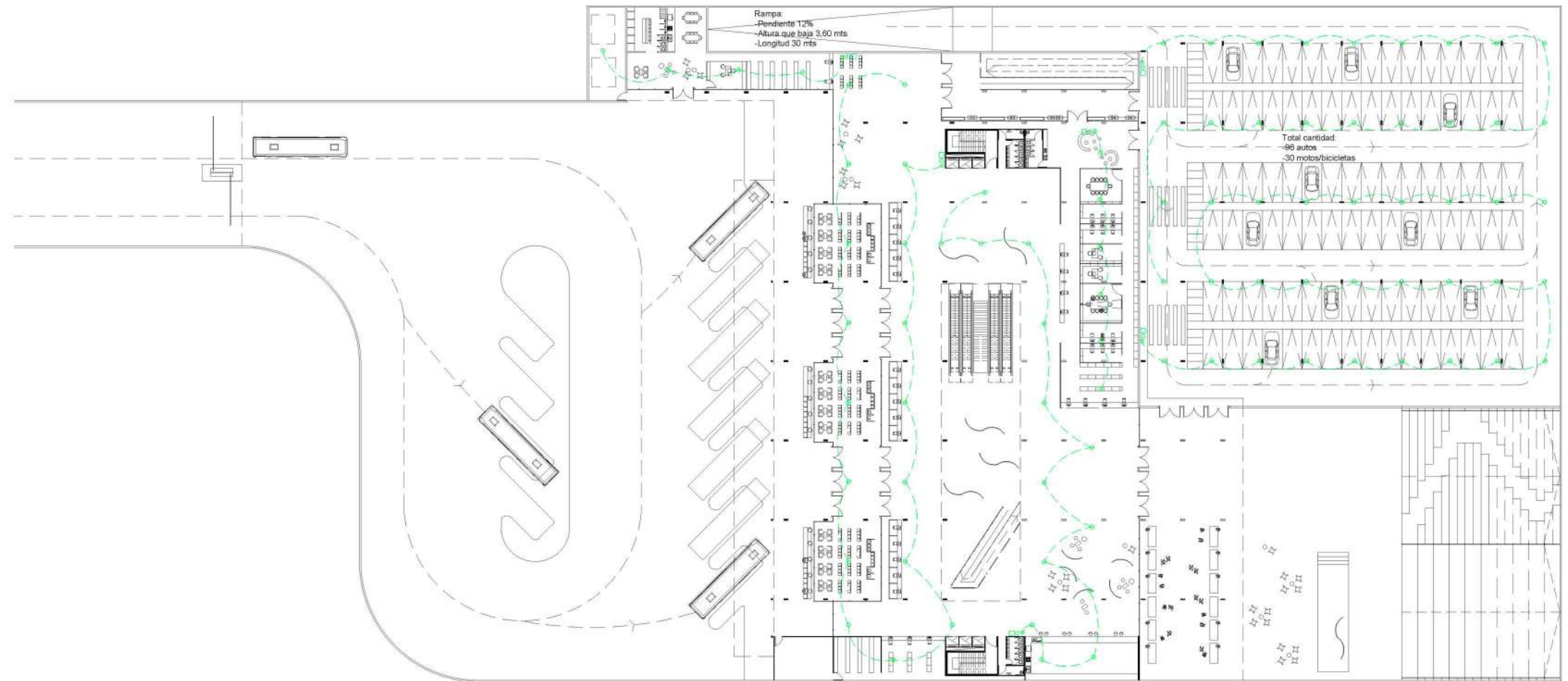
Planta nivel - 3,60 mts
