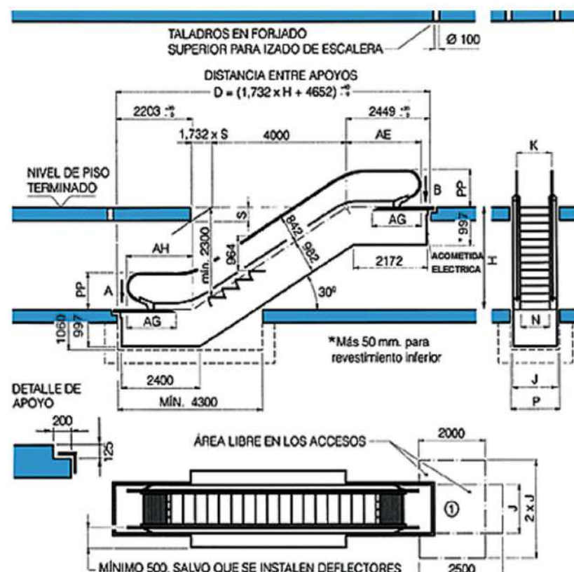
Escalera mecánica
