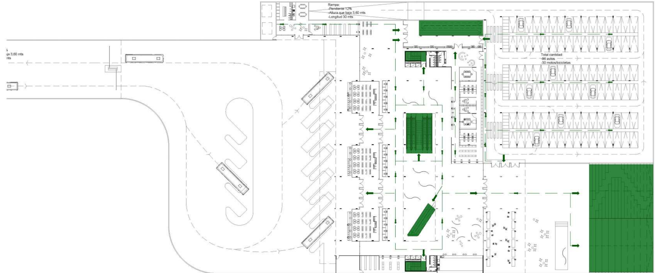
Planta nivel - 3,60 mts
