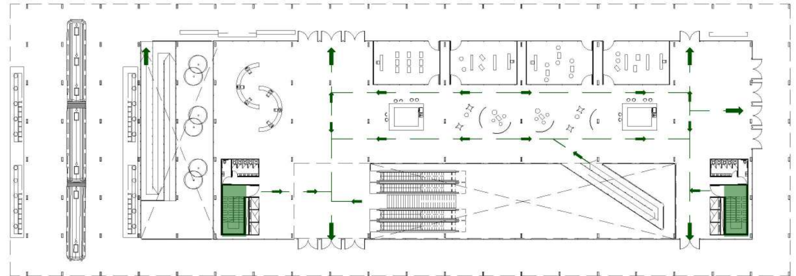
Planta nivel + 2,00 mts
