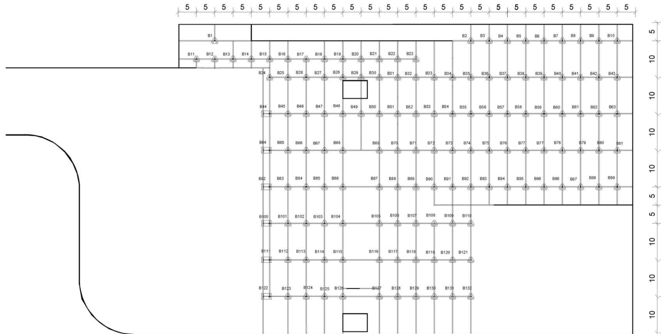
Planta de fundaciones nivel -3,60 mts
