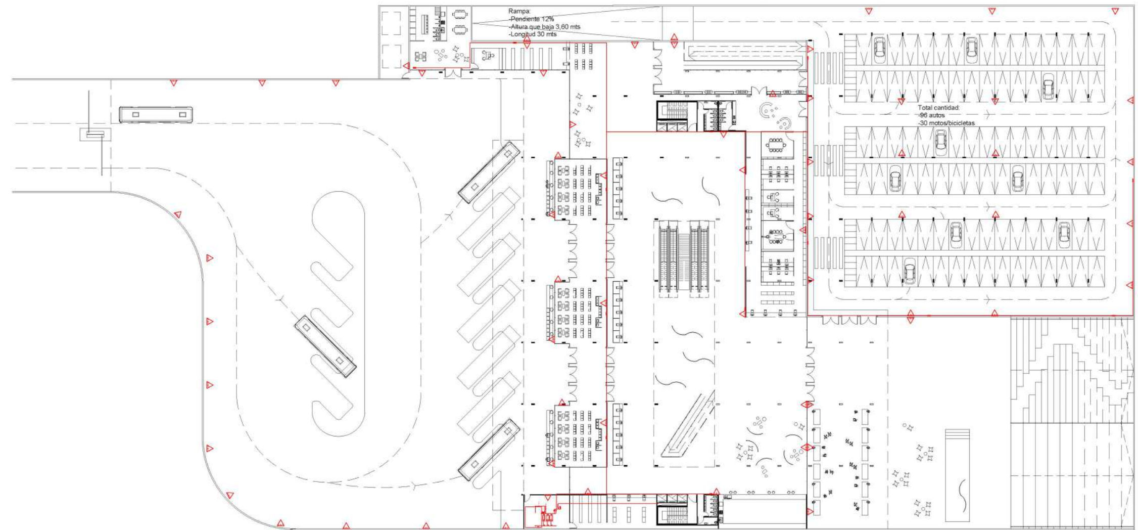
Planta nivel - 3,60 mts
