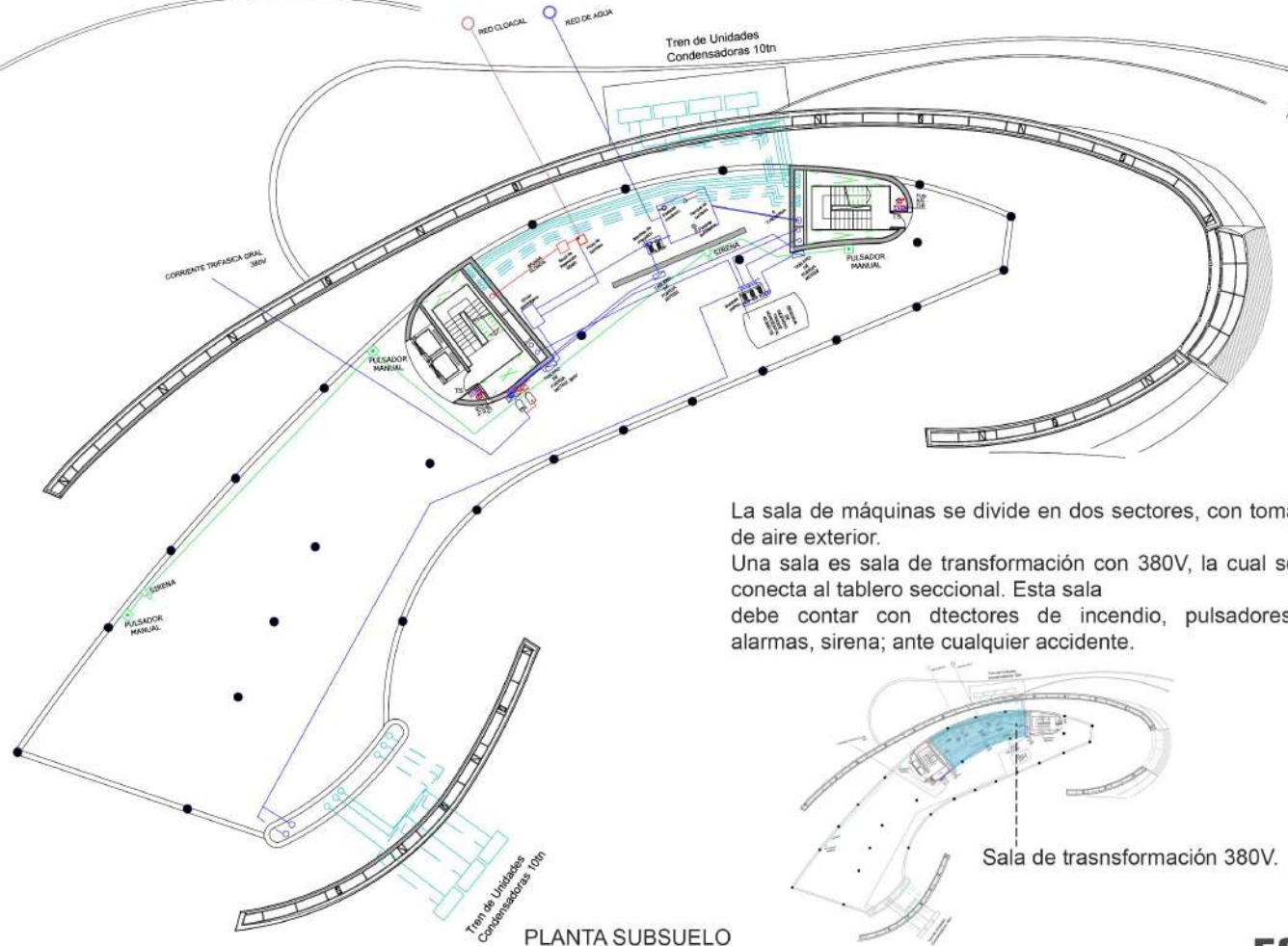
PLANTA SUBSUELO
