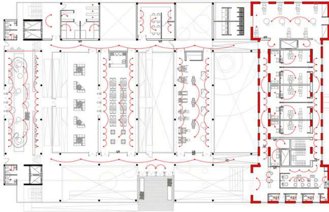
PLANTA -4.5 Centro de Diagnóstico y Tratamiento
