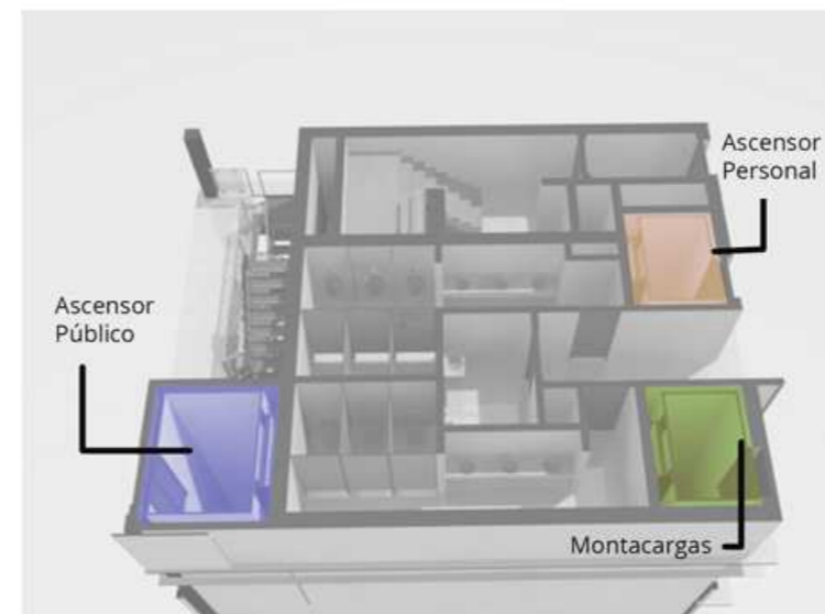
Detalle de ubicación de ascensores y montacargas en núcleo de servicios
