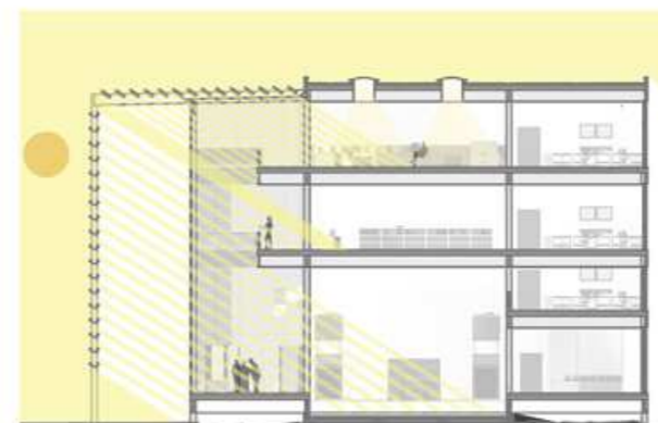
Gráfico en corte de acond. térmico pasivo en invierno Rayos solares a 30°
