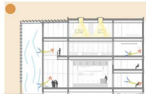
Gráfico en corte de acond. térmico pasivo en verano Rayos solares a 78°
