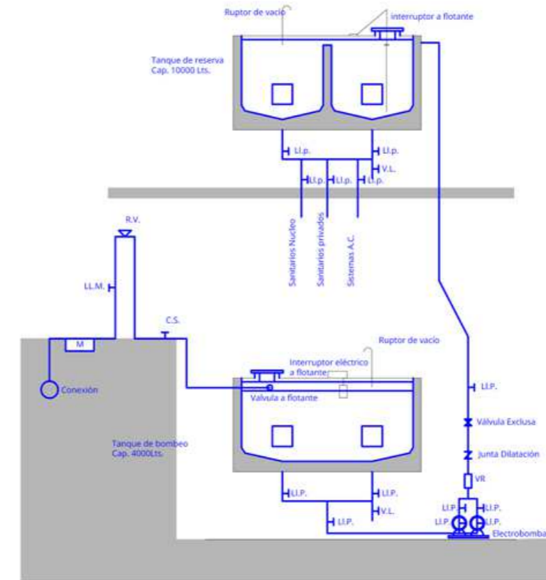
Esquema en corte de Provisión de Agua Fría
