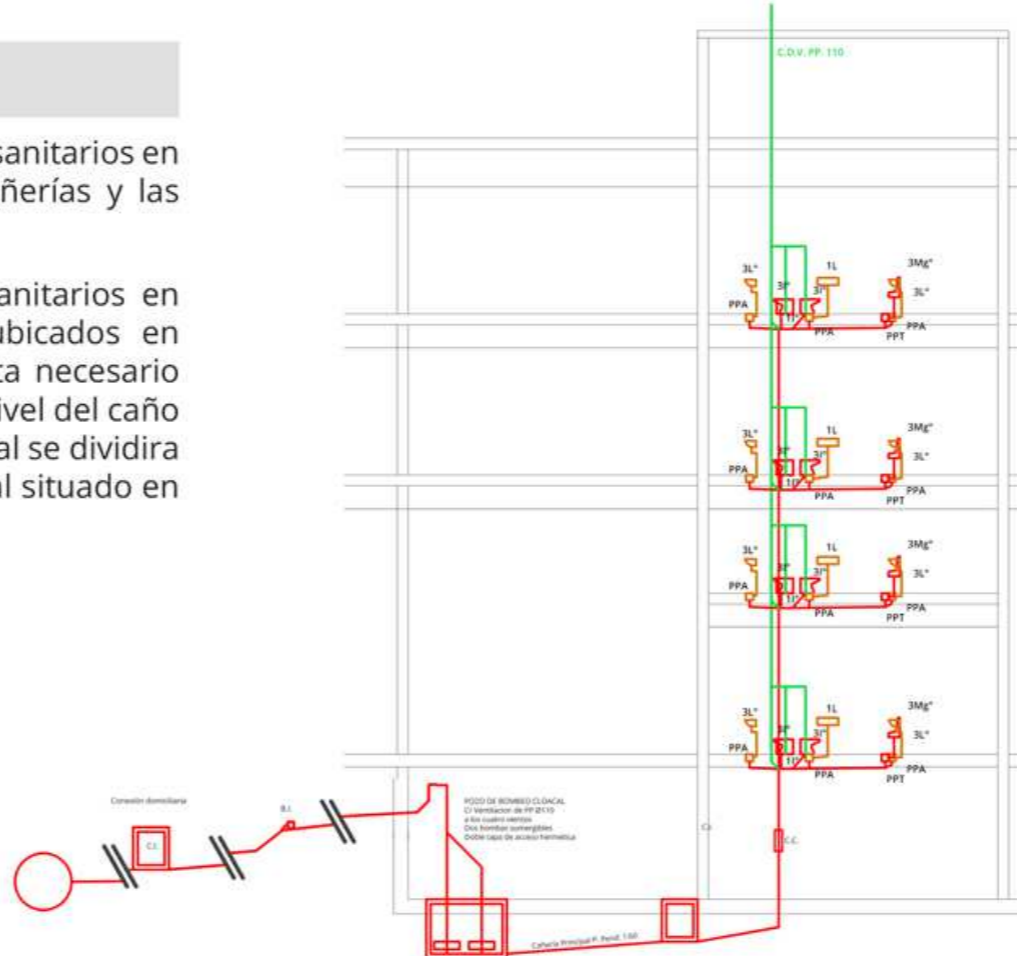
Detalle en corte de desagüe cloacal
