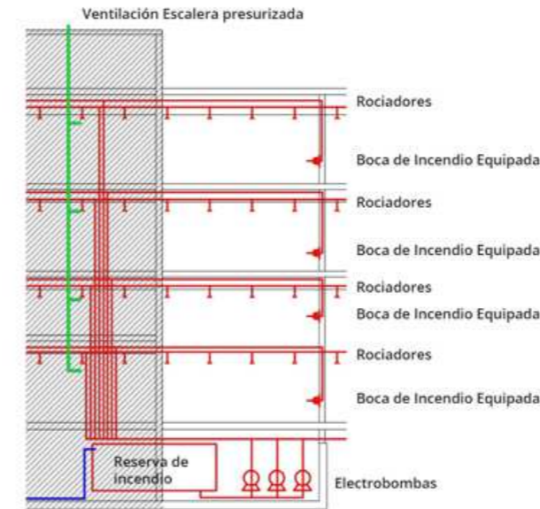
Esquema en corte de abastecimiento de agua presurizado en sistema contra incendios
