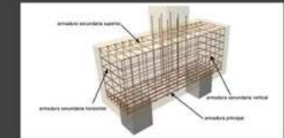
Doble pilote con cabezal de Hormigón
