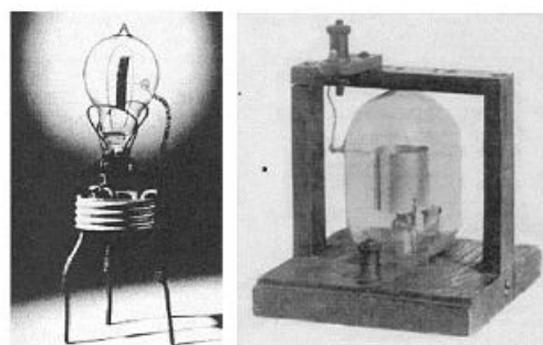
Válvulas de Fleming, con filamentos de carbón. 1904-1908
