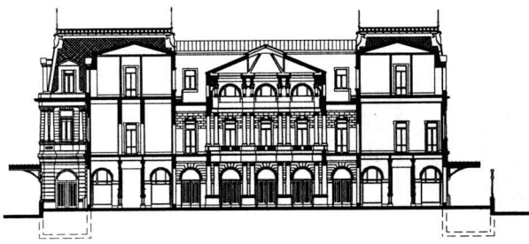
Pasaje Dardo Rocha. Corte transversal
