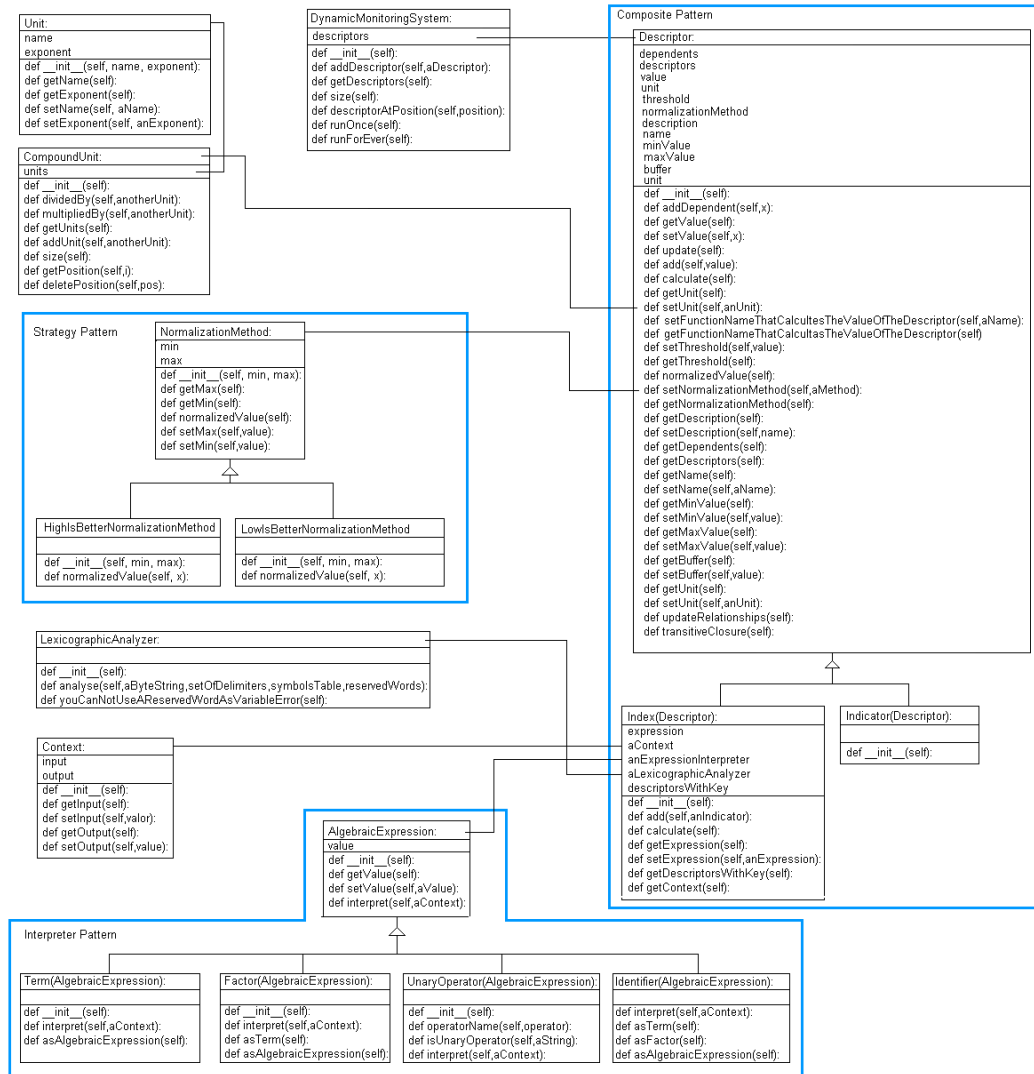
Figura 6. Framework para el desarrollo de modelos sistémicos basados en índices e indicadores cuantitativos.
