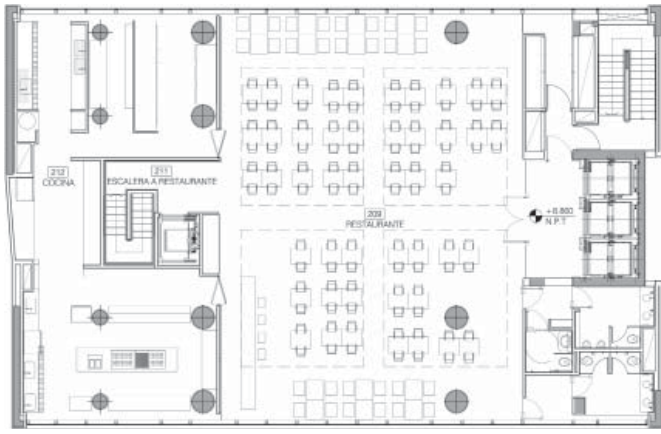
PLANTA RESTAURANTE + 8.86
