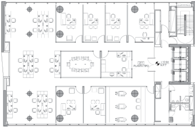
PLANTA TIPO 1º, 3º, 4º, 5º, 9º, 10º, 11º y 12º PISO
