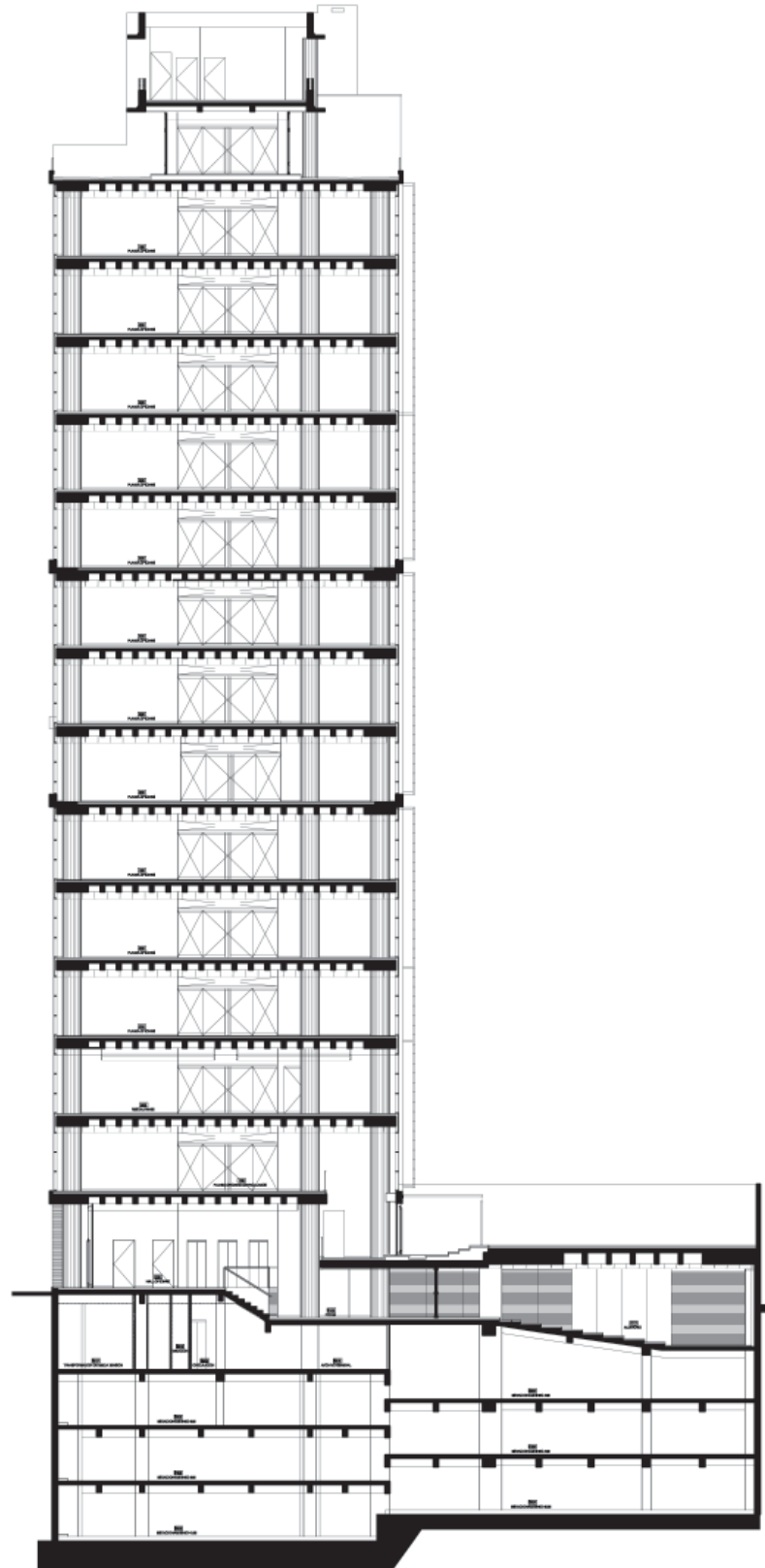
CORTE B-B
