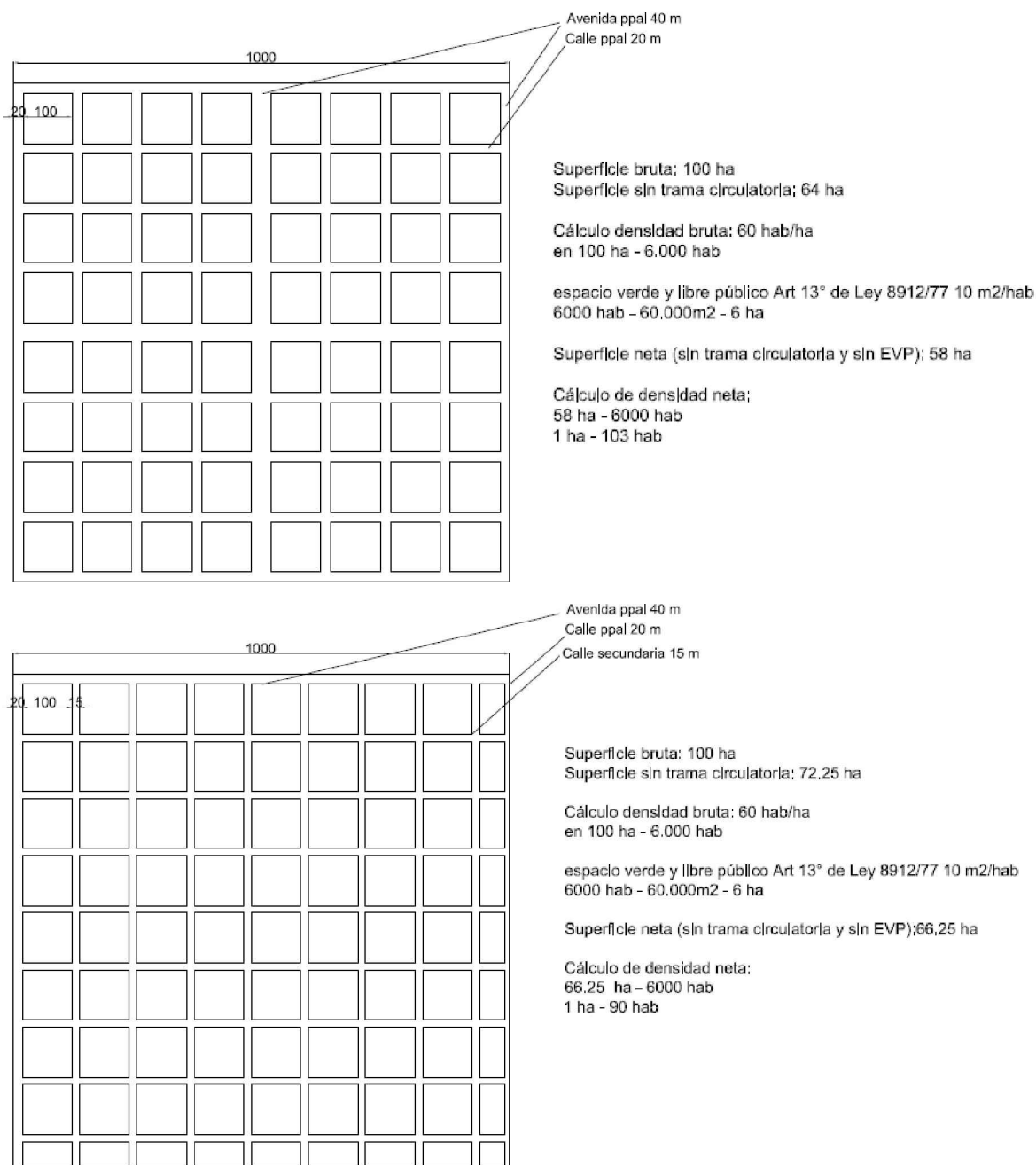
FIGURA N°18: CÁLCULO DE LA DENSIDAD NETA EN RELACIÓN A LA DENSIDAD BRUTA NORMADA POR EL DTO. 3202/06. ALTERNATIVAS SEGÚN POSIBLES ANCHOS DE CALLE Elaboración propia
