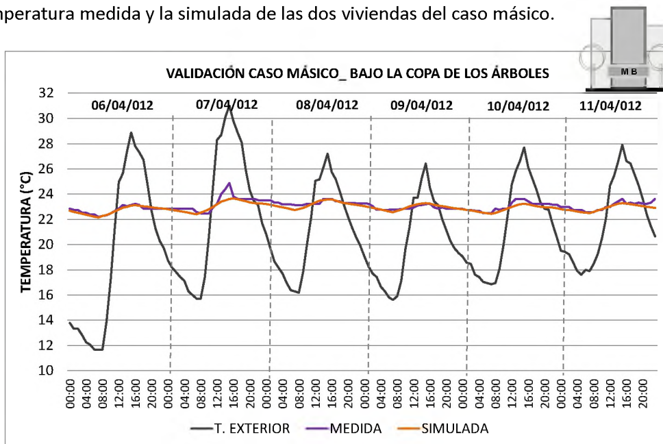
Figura V.3. Ajuste y validación del caso másico bajo la copa en Energy Plus
