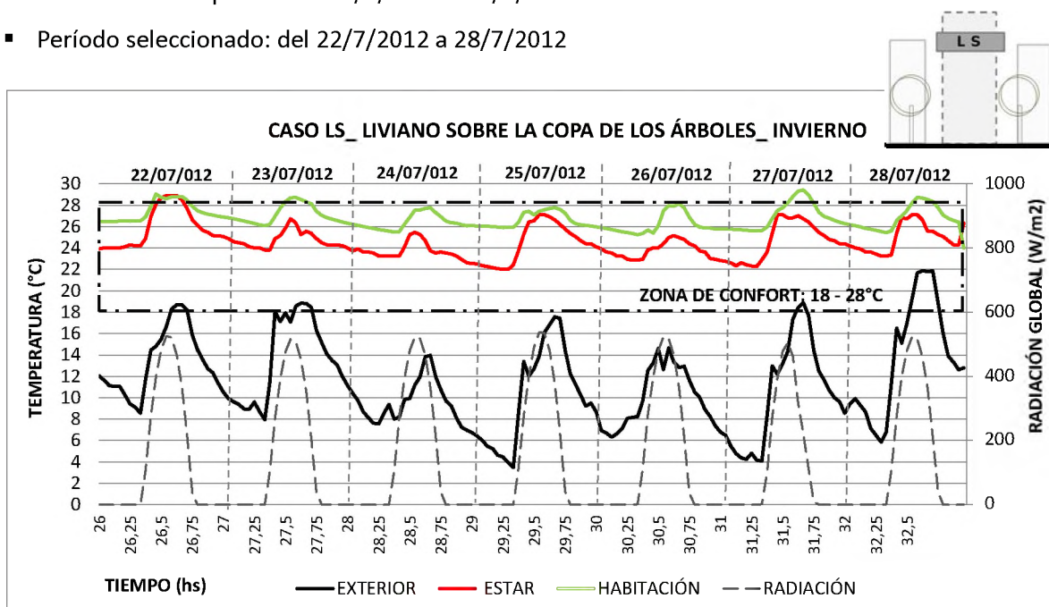
Figura IV.37. Temperatura exterior e interiores en invierno de la vivienda liviana sobre la copa
