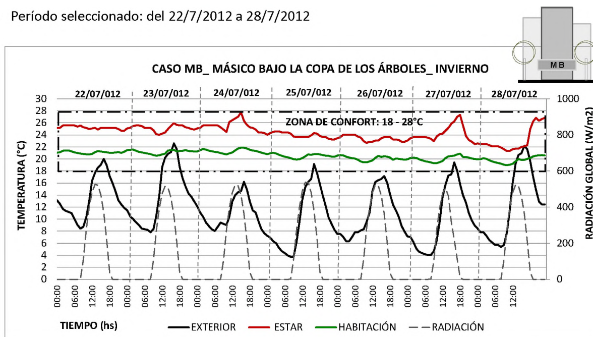
Figura IV.19. Temperatura exterior e interiores en invierno de la vivienda másica bajo la copa
