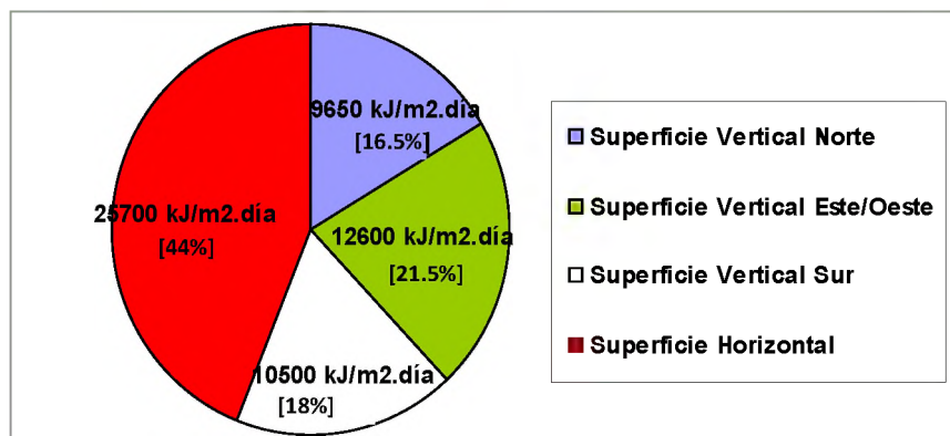
Figura II.7. Radiación incidente diaria en verano (diciembre) para las distintas superficies verticales y para la superficie horizontal
