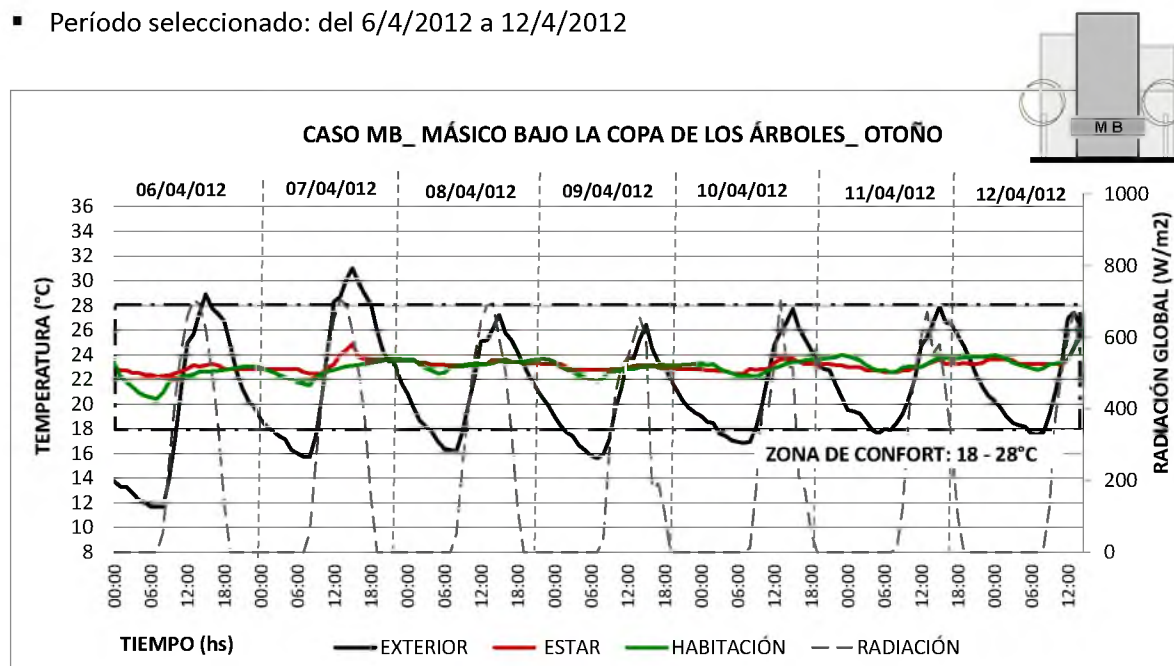
Figura IV.18. Temperatura exterior e interiores en otoño de la vivienda másika bajo la copa
