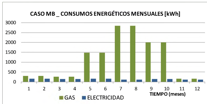
Figura IV.21. Consumos mensuales de la vivienda másica bajo la copa de los árboles
