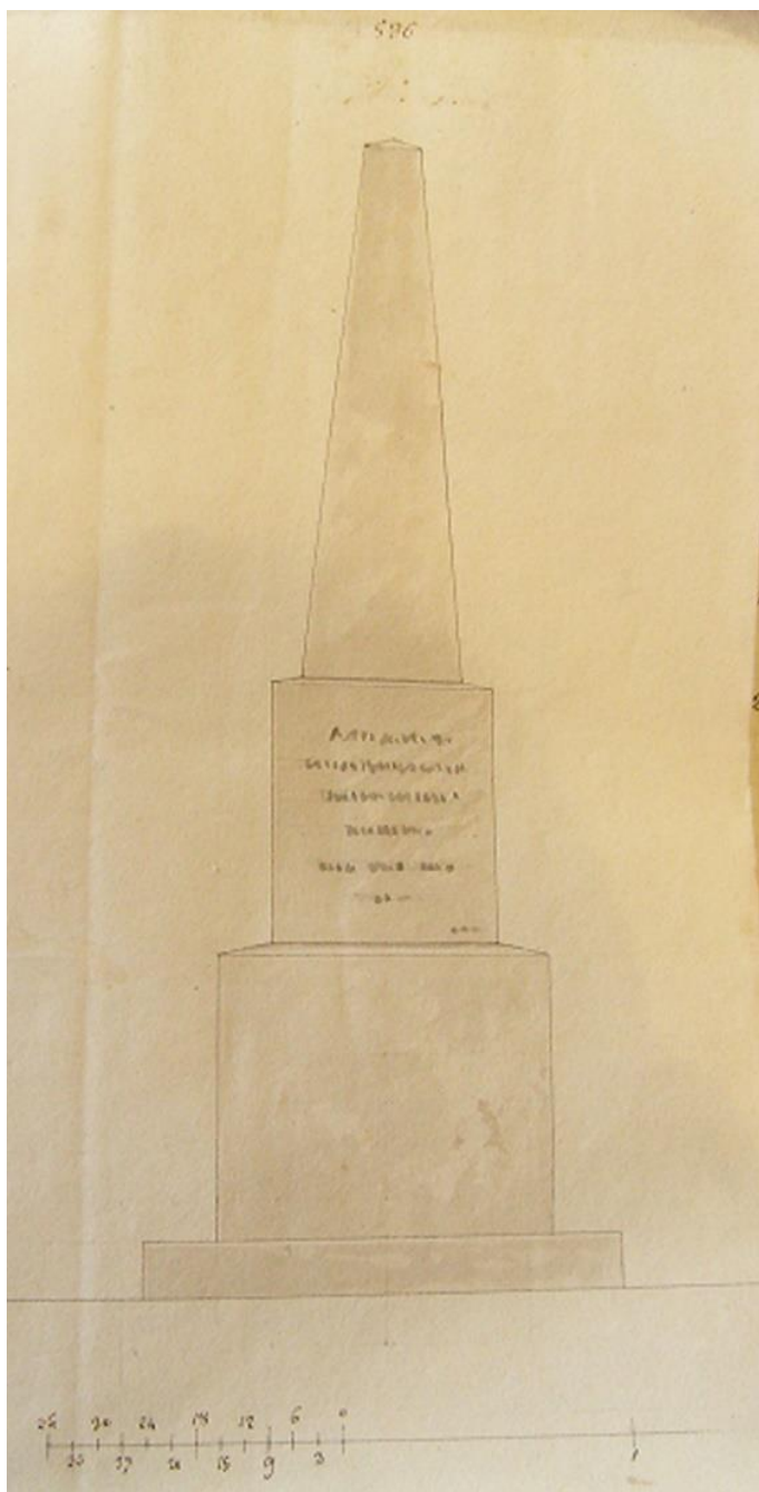
Figura 13. Plano del Ingeniero Carlo Zucchi para el monumento fúnebre en honor a Antonio Saenz. AGN, Sala X, 36-4-5, 1831.
