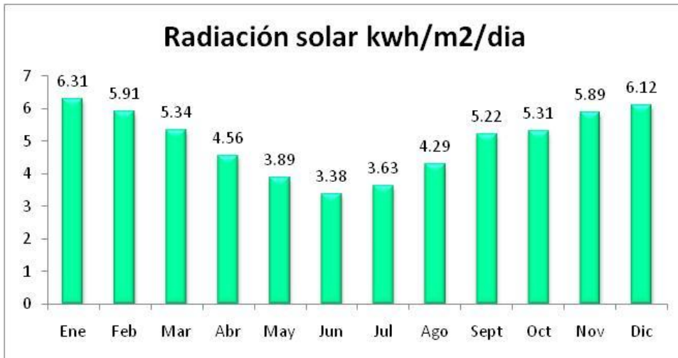
Gráfico 67. Radiación solar mensual (kWh/m2día) para una inclinación de 34° (LATITUD 34,4)
