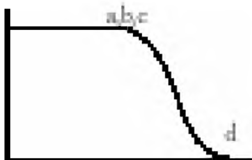
Figura 44: Función sigmoideal decreciente, para Ar el valor de a=100\text{m} y d=1000\text{m} , para Pe a=20\% y d=15\%
