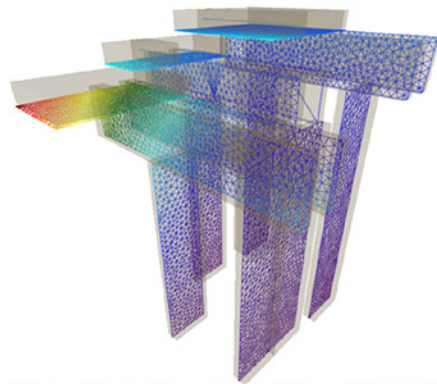
distribución de tensiones de Von Mises
