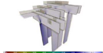
esfuerzo axil en elementos verticales
