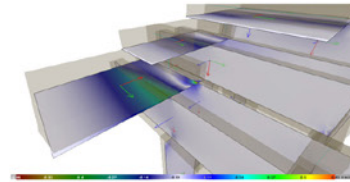
esfuerzo axil longitudinal en vigas
