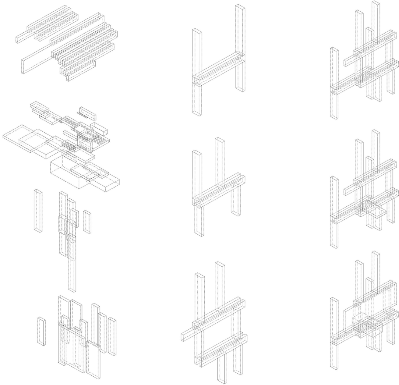
PROCESO GENERATIVO INTERNO. Materias Desestratificadas. Sistemas de piezas y componentes. Detalle de los componentes en axonométrica (despiece)
