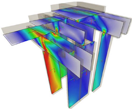
distribución de tensiones de Von Mises
