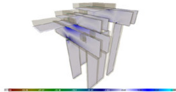
esfuerzo axil en elementos verticales
