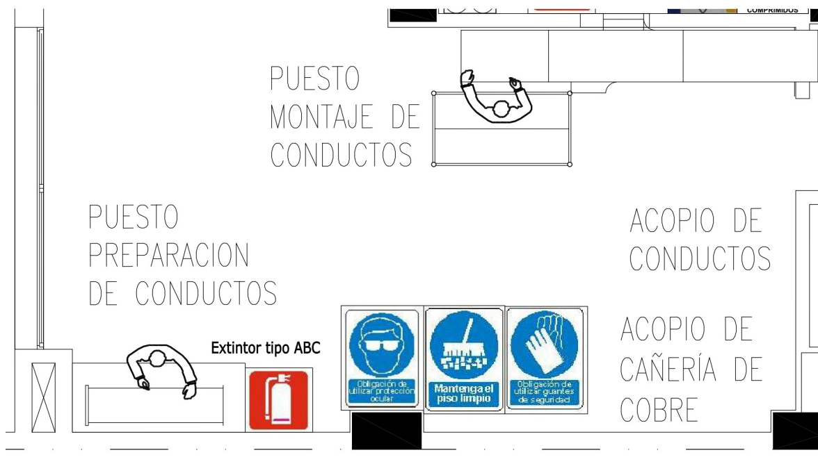
Figura 12. Puesto de trabajo: preparación, ajustes, realización de agujeros para derivaciones, aislación de conductos de chapa galvanizada.
