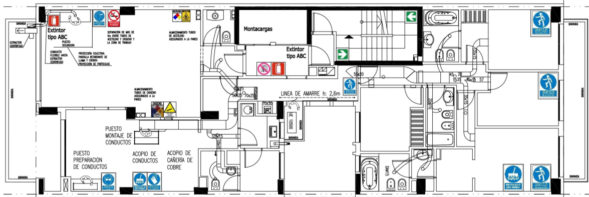
Figura 5. Planta tipo utilizando equipos separados. Con puestos de trabajo.
