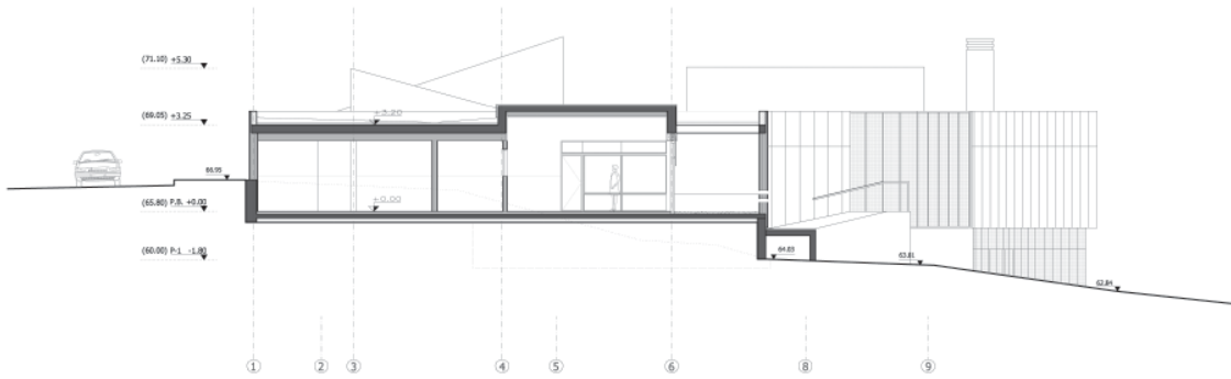
SECCIÓ A-A
