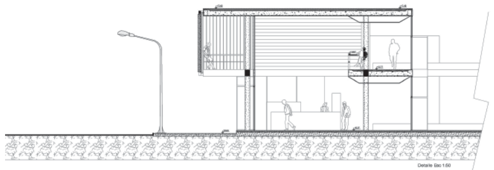
Detalle Esc 1:50
