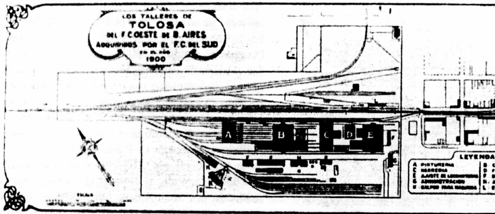
Figura 2: Planta general de los talleres ferroviarios de Tolosa. Año 1884. Ing. Otto Krause. Archivo Histórico de la Provincia de Buenos Aires.
