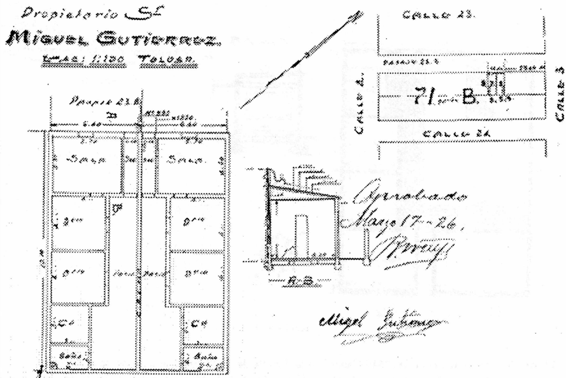
Figura 1: Primeras transformaciones tipológicas: el w.c. fue reemplazado un baño a expensas de la reducción de la cocina y la galería fue eliminada para agrandar el patio lateral. Archivo de la Dirección de Obras Particulares de la Municipalidad de La Plata
