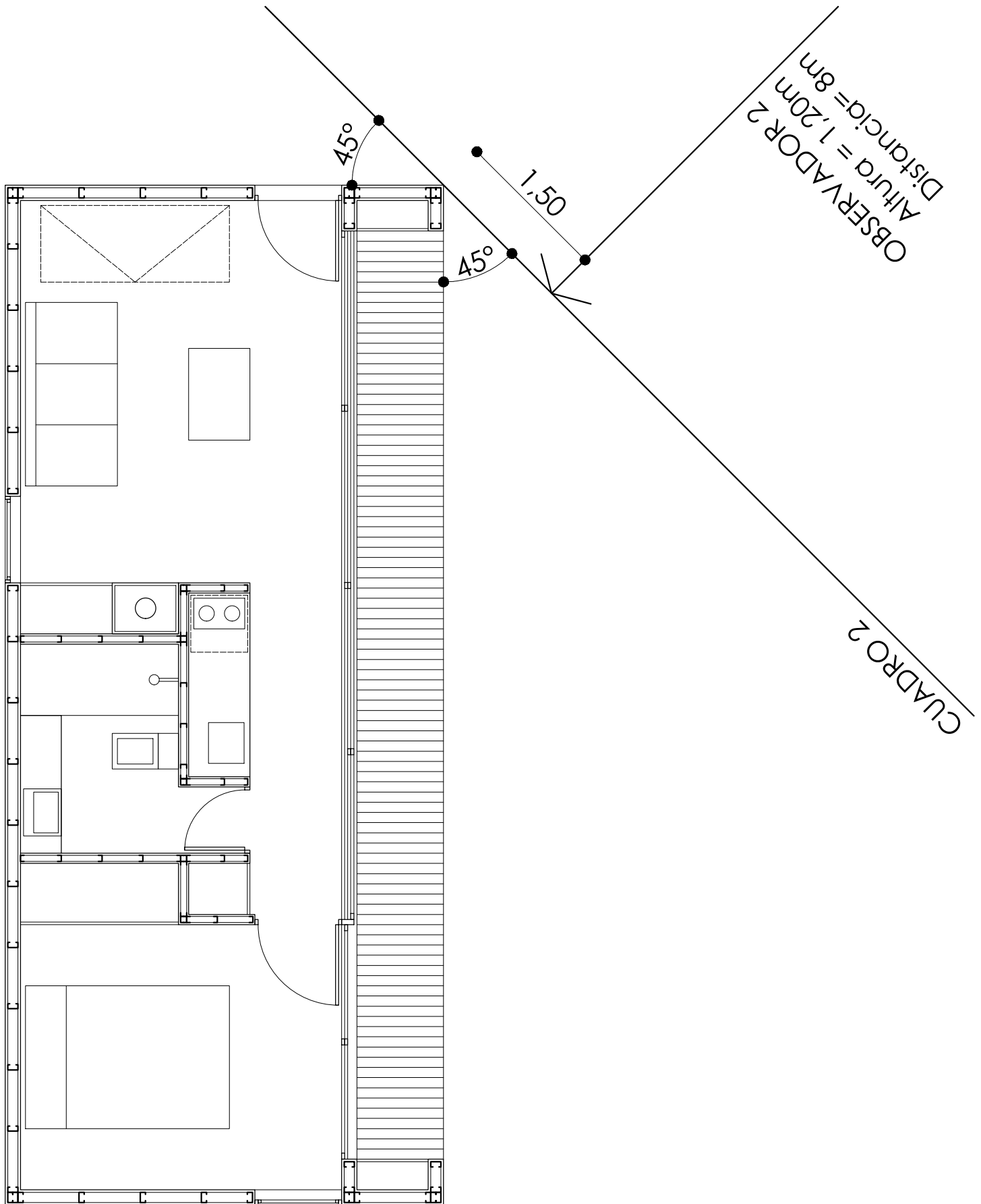
PLANTA 1:50
