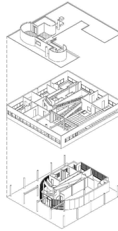
Perspectiva Axonométrica Isométrica Explotada
