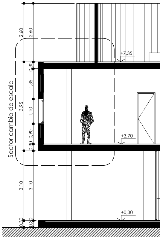
Ville Savoye | SECTOR CORTE A-A ESC 1:100
