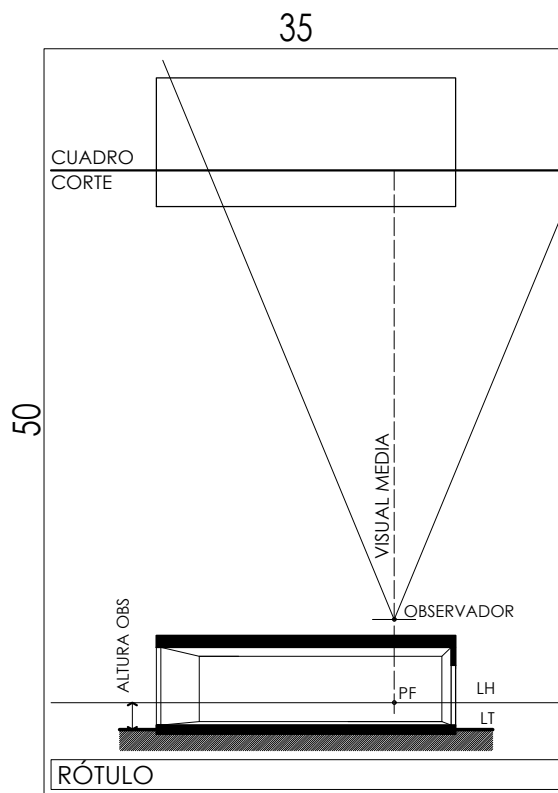
CASO 2 CORTE PERSPECTIVADO A UN PUNTO DE FUGA
