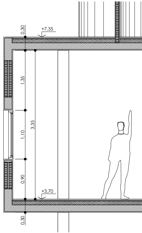
Ville Savoye | SECTOR CORTE ESC 1:50
