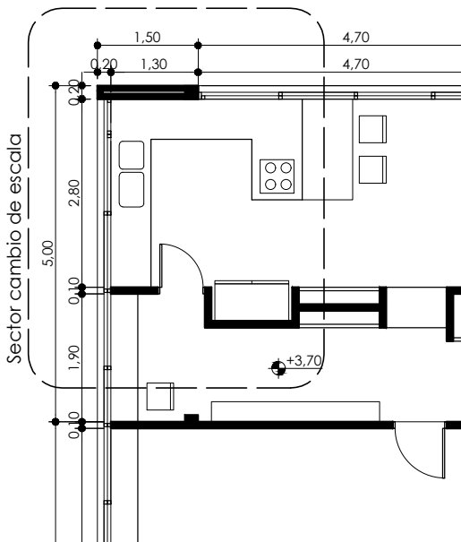
Ville Savoye | SECTOR PLANTA ESC 1:100
