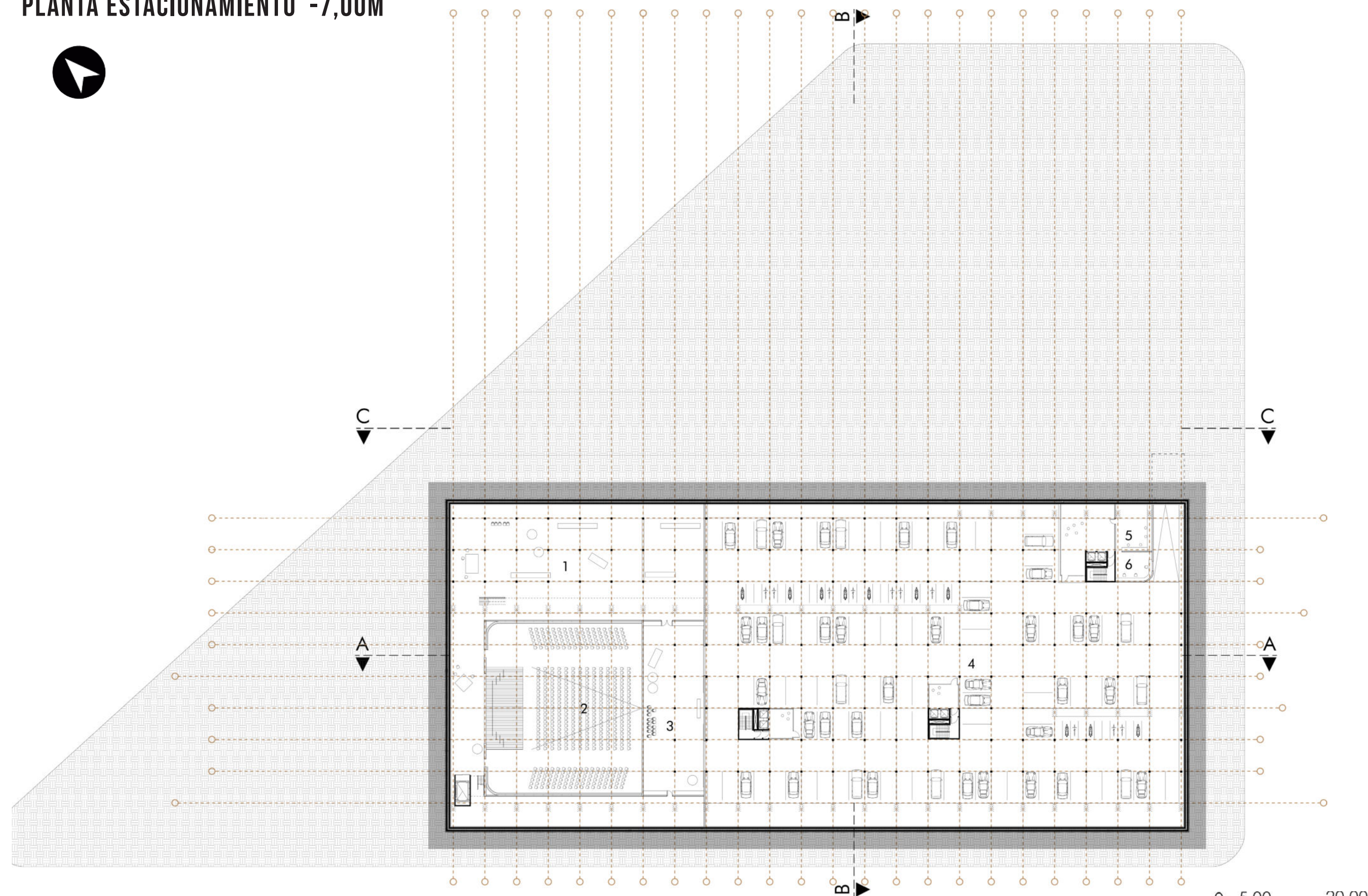
1 - Taller de escenografía / 2 - Sala de espectáculos / 3 - Deposito / 4 - Estacionamiento / 5 - Sala de monitoreo / 6 - Control de acceso
