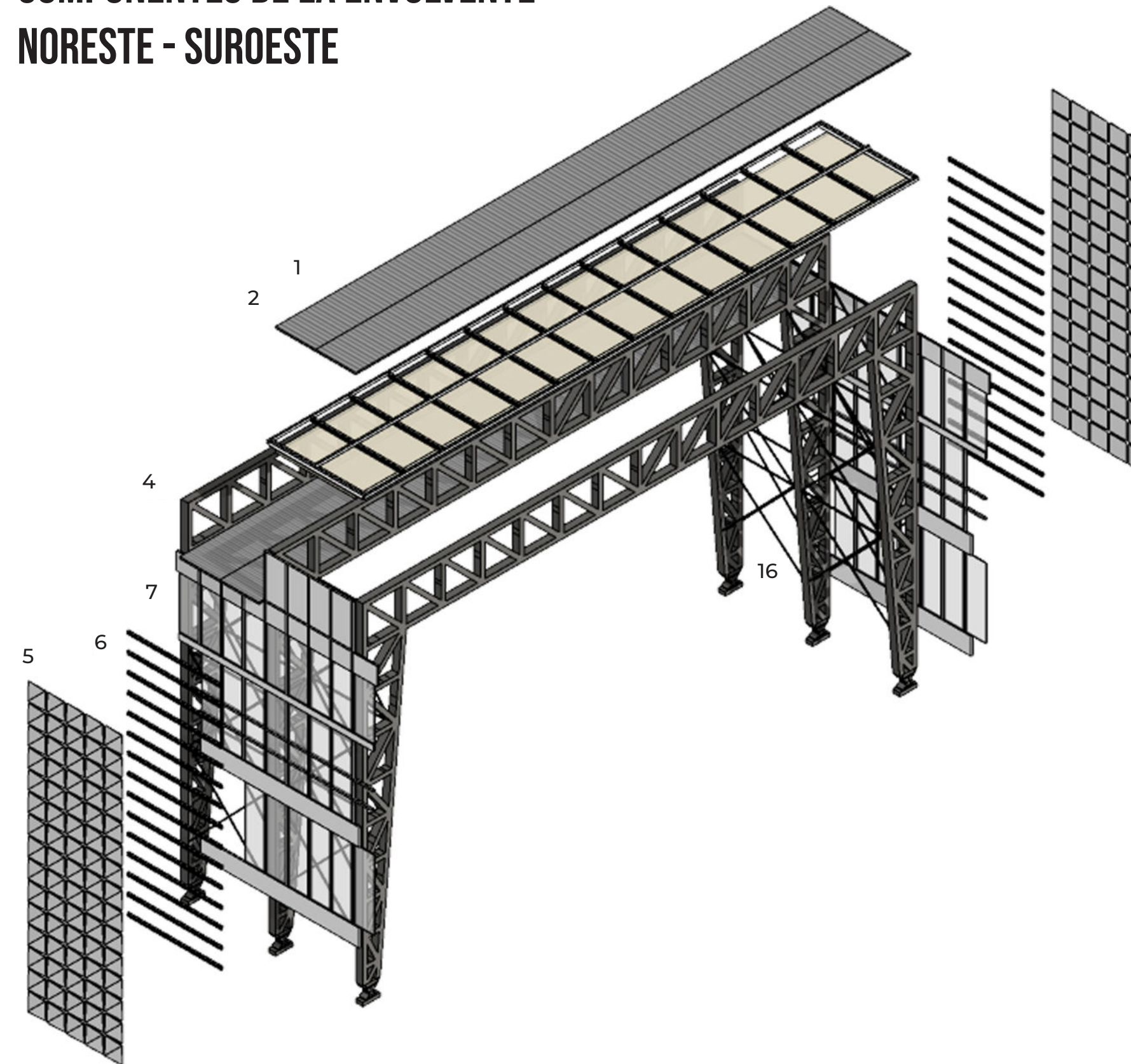
1 - Paneles fotovoltaicos / 2 - Cubierta de chapa con pendiente / 3 - Aislación termica lana de vidrio / 4 - Pórtico metálico reticulado / 5 - Paneles de chapa microperforados / 6 - Perfiles subestructura de paneles / 7 - Piel de vidrio (Carpintería de aluminio + DVH) / 8 - Paneles de entrepiso autoportantes PUR / 9 - Vigas reticuladas / 10 - Tensores metálicos / 11 - Barandas de seguridad metálicas / 12 - Tabique de contención + cámara de aire + ladrillo común / 13 - Vínculo metal hormigón / 14 - Estructura de hormigón armado / 15 - Contrapiso + aislación / 16 - Cruces de San Andrés
