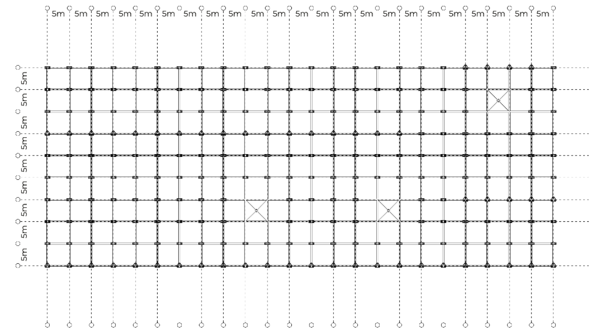
PRIMER ENTREPISO (IN SITU)
