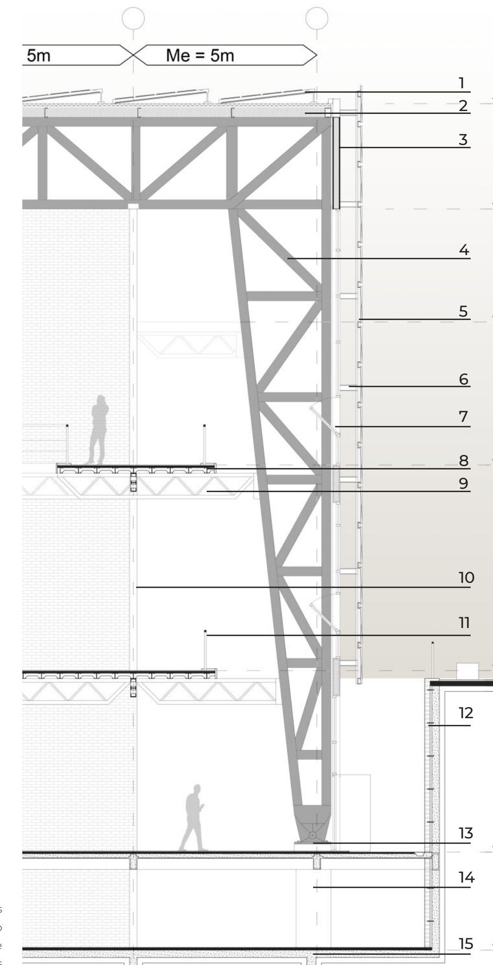
1 - Paneles fotovoltaicos / 2 - Cubierta de chapa con pendiente / 3 - Aislación termica lana de vidrio / 4 - Pórtico metálico reticulado / 5 - Paneles de chapa microperforados / 6 - Perfiles subestructura de paneles / 7 - Piel de vidrio (Carpintería de aluminio + DVH) / 8 - Paneles de entrepiso autoportantes PUR / 9 - Vigas reticuladas / 10 - Tensores metálicos / 11 - Barandas de seguridad metálicas / 12 - Tabique de contención + cámara de aire + ladrillo común / 13 - Vínculo metal hormigón / 14 - Estructura de hormigón armado / 15 - Contrapiso + aislación / 16 - Cruces de San Andrés
