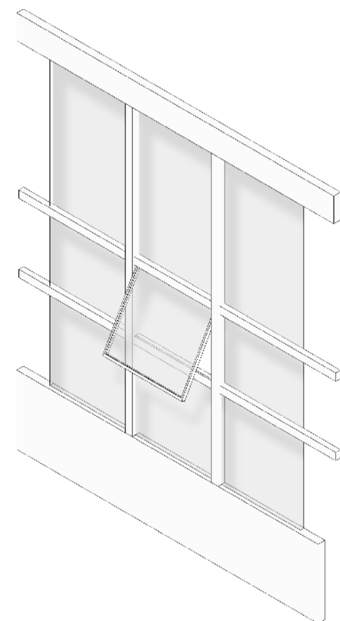
ACCIONAMIENTO DE VENTANAS
