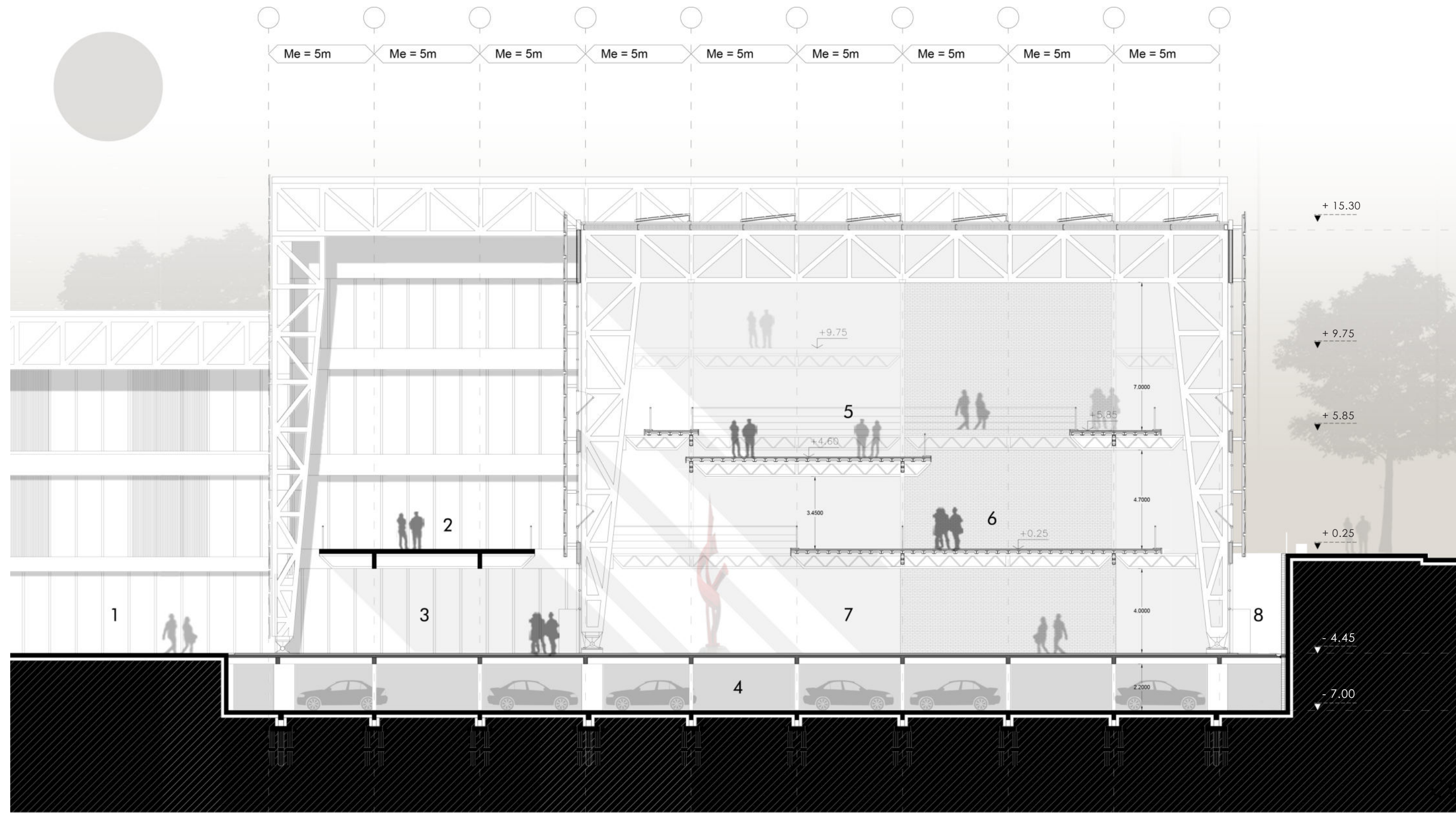
1 - Plaza de acceso / 2 - Acceso / 3 - Acceso / 4 - Estacionamiento / 5 - Sala de expo permanente / 6 - Sala de expo temporal / 7 - Hall y expo / 8 - Patio
