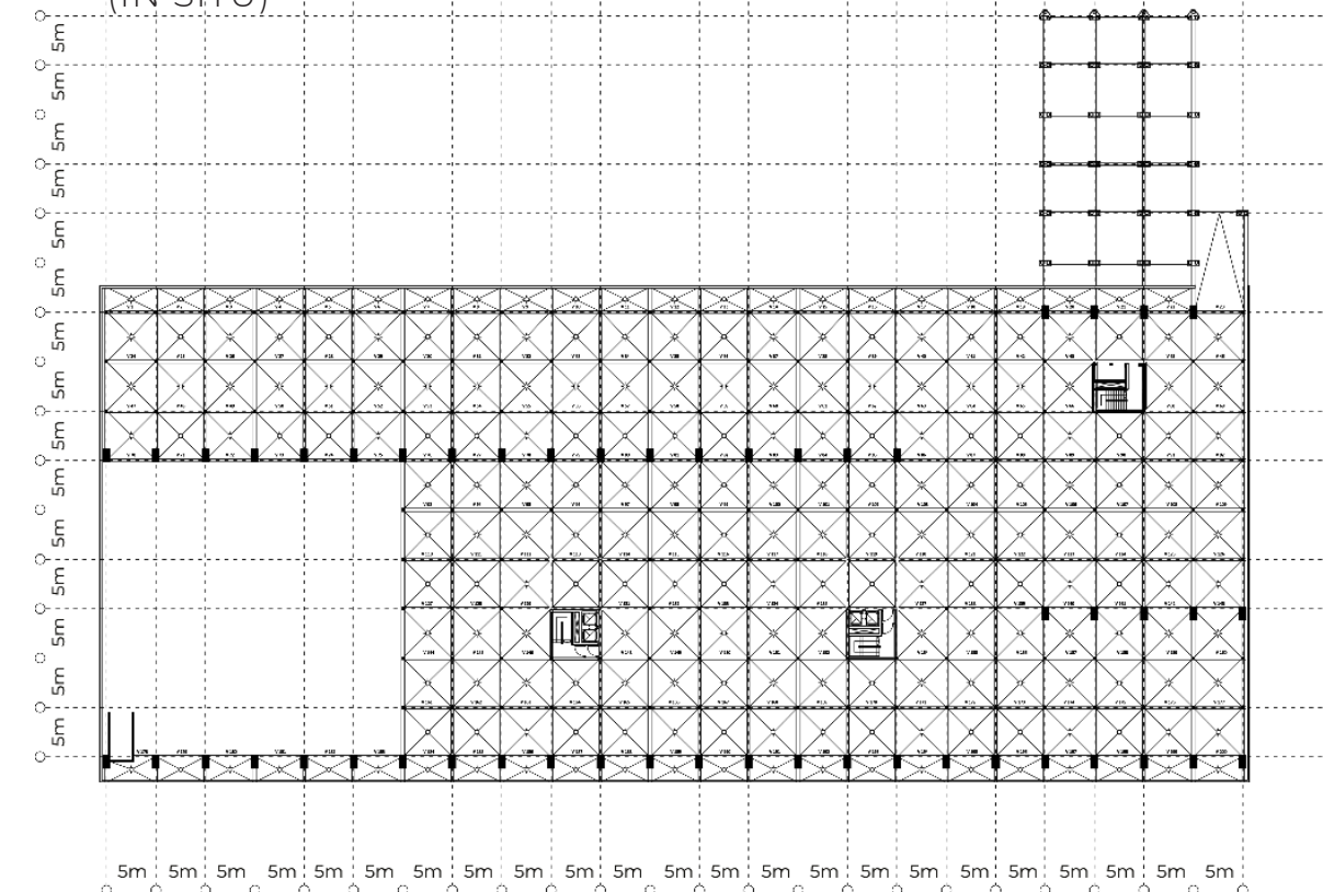
PRIMER ENTREPISO (IN SITU)
