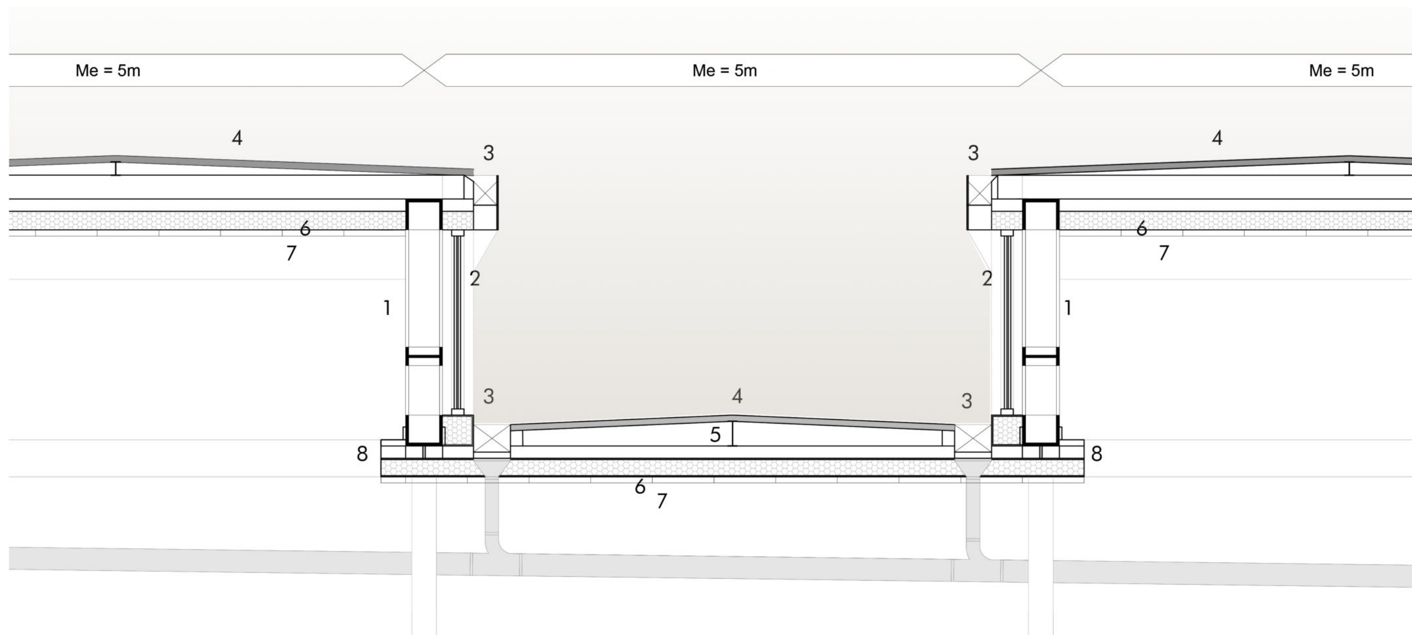
1 - Dintel pórtico metalico reticulado / 2 - Carpinteria de PVC con doble vidrio hermetico / 3 - Desagües pluviales con desembocadura en embudos de recoleccion de agua / 4 - Cubierta metalica con pendiente / 5 - Estructura secundaria de la cubierta - Perfil HEA / 6 - Aislacion termo-acustica lana de vidrio / 7 - Revestimiento metalico chapa lisa / 8 - Perfil de vinculo de la estructura con la cubierta suspendida
