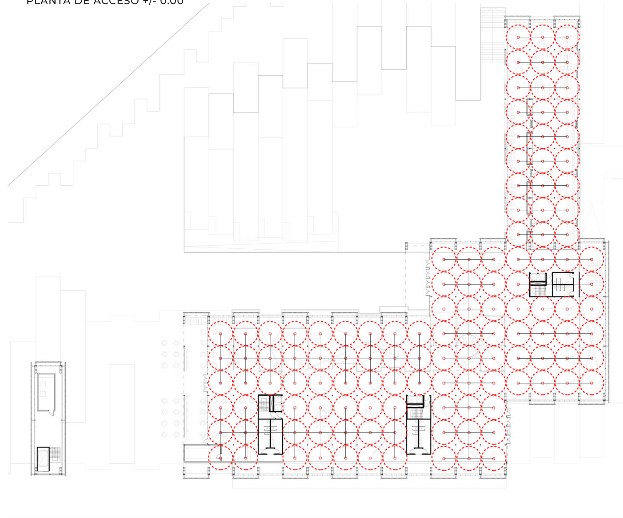
PLANTA DE ACCESO +/- 0.00
