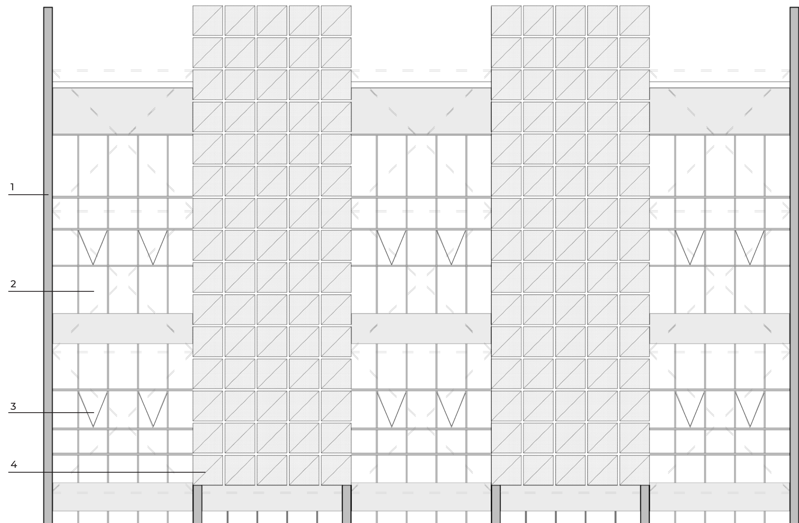
1 - Porticos metálicos / 2 - Paños fijos DVH con carpintería de aluminio / 3 - Ventanas con accionamiento tipo banderola con DVH / 4 - Paneles de chapa microperforada
