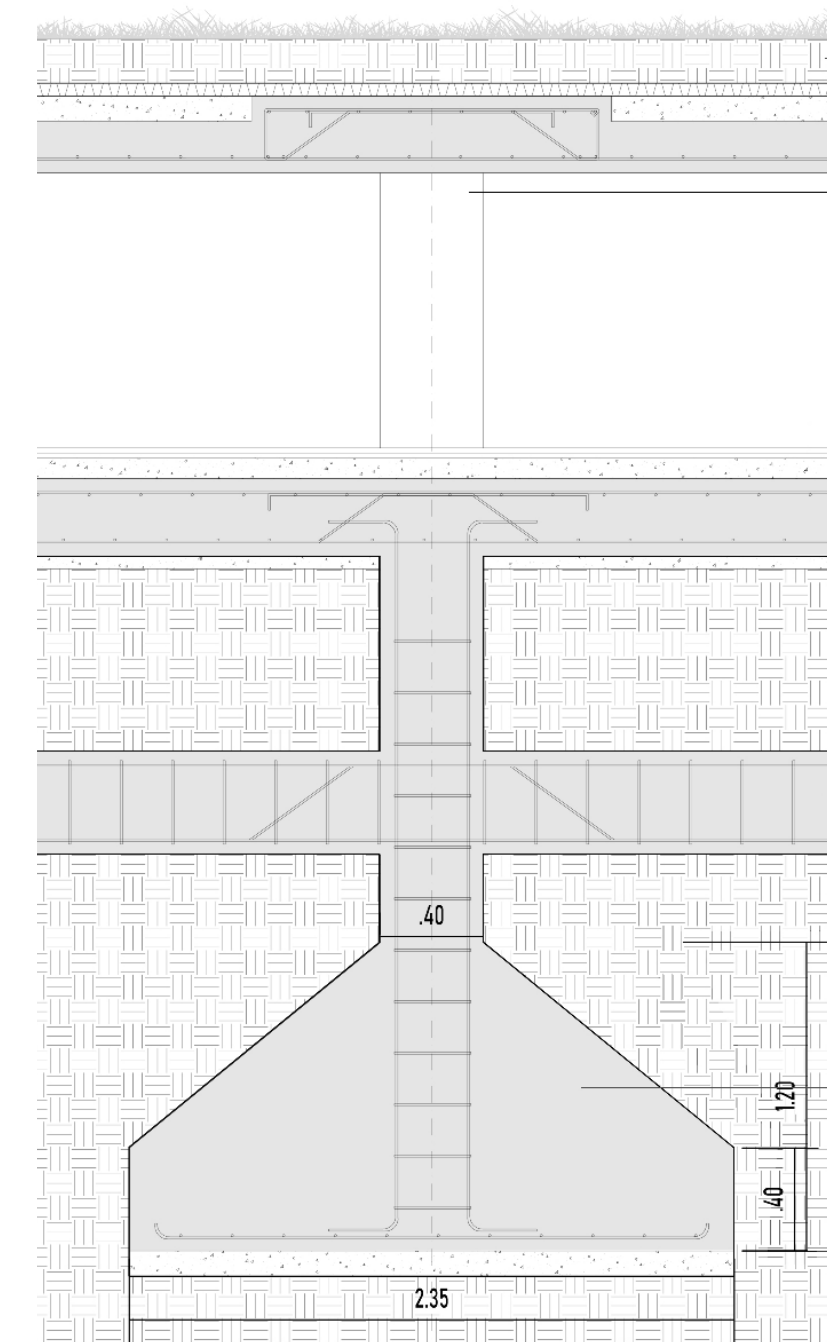
01 Sustrato natural 02 Contrapiso de cascote con poliestireno expandido 03 Tronco de base 04 Base de HPA 05 Hormigón de limpieza 06 Film de polietileno expandido 200 micrones -Aislante Hidrófugo-
