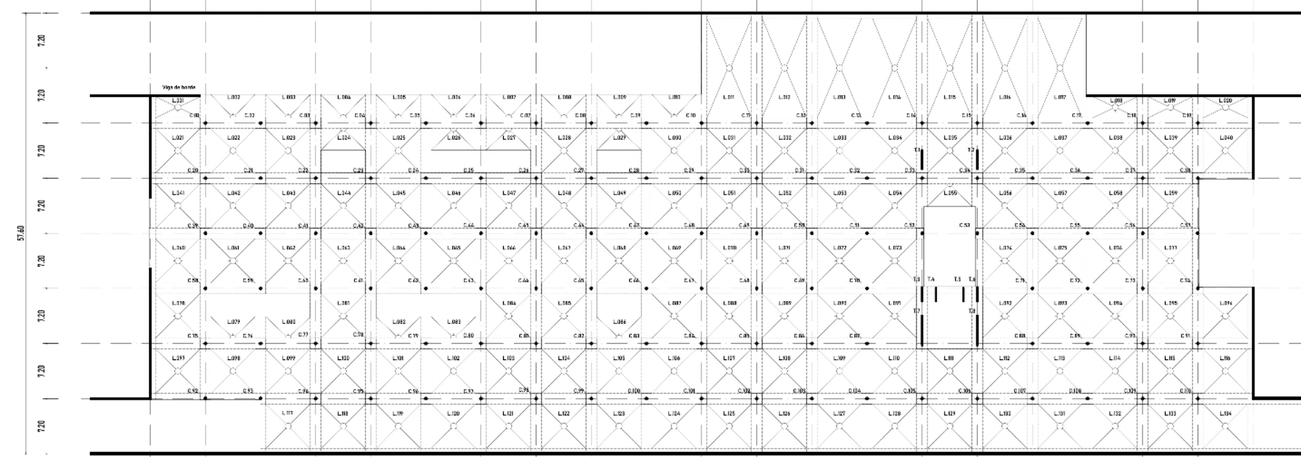
Planta Estructural nivel 0.00. Entrepiso sin vigas postesado, espesor 0.20m que aumenta a 0.30m en forma de capiteles invertidos.
