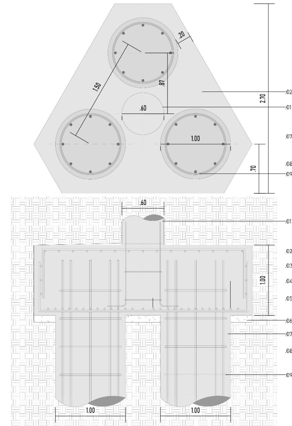
01 Columna de HPA diam. 0.40m 02 Cabezal o encapado de HPA 03 Armadura plano superior 04 Armadura principal 05 Armadura plano inferior 06 Hormigón de limpieza 07 Pilote de 1.00m de diámetro, aumenta a 1.50m 08 Armadura principal pilote 09 Estribos
