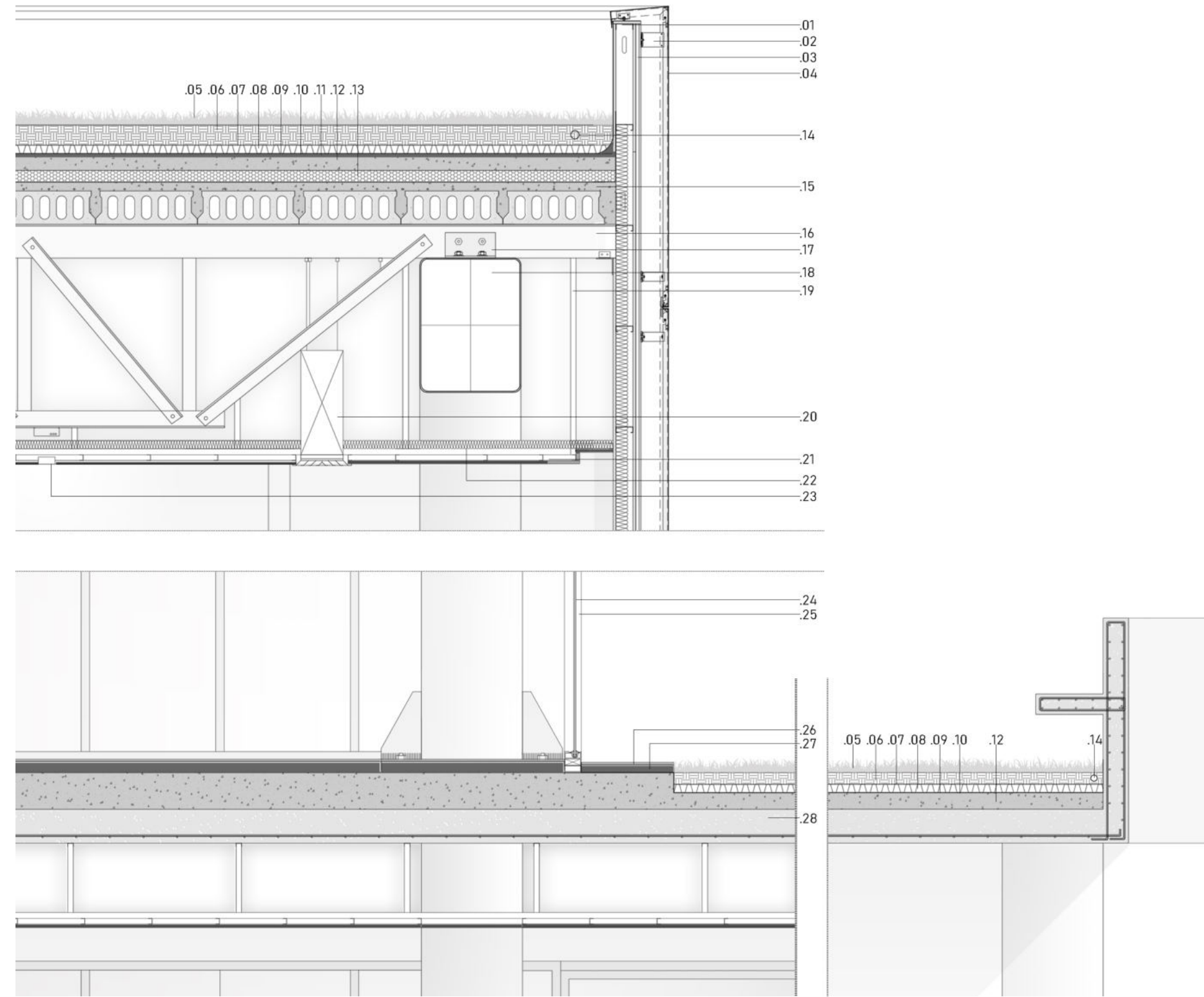
01 Estructura de steel 02 Soporte de pared 03 Placa OSB 04 Panel Alucobond 05 Cesped 06 Sustrato 07 Manto geotextil 08 Placa termoadesiva 09 Barrera anti-raiz 010 Membrana asfáltica 011 Carpeta 012 Contrapiso 013 Poliestireno expandido 014 Desague de cubierta 015 Losa alveolar y capa de compresión 016 Viga reticulada perfiles "L" 017 Anclaje metálico abulonado 018 Cordón superior de viga reticulada de acero 019 Vela rígida, estructura auxiliar cielorraso 020 Conducto de A-A 021 Placa cielorraso 022 Material fonoabsorbente 023 Iluminación 024 DVH 025 Carpintería de aluminio 026 Piso cerámico 027 Carpeta 028 Losa de entrepiso sin vigas.
