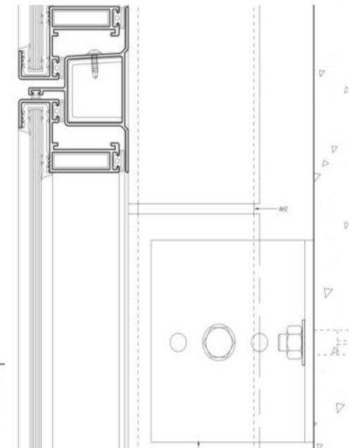
Detalle perfil-perfil
