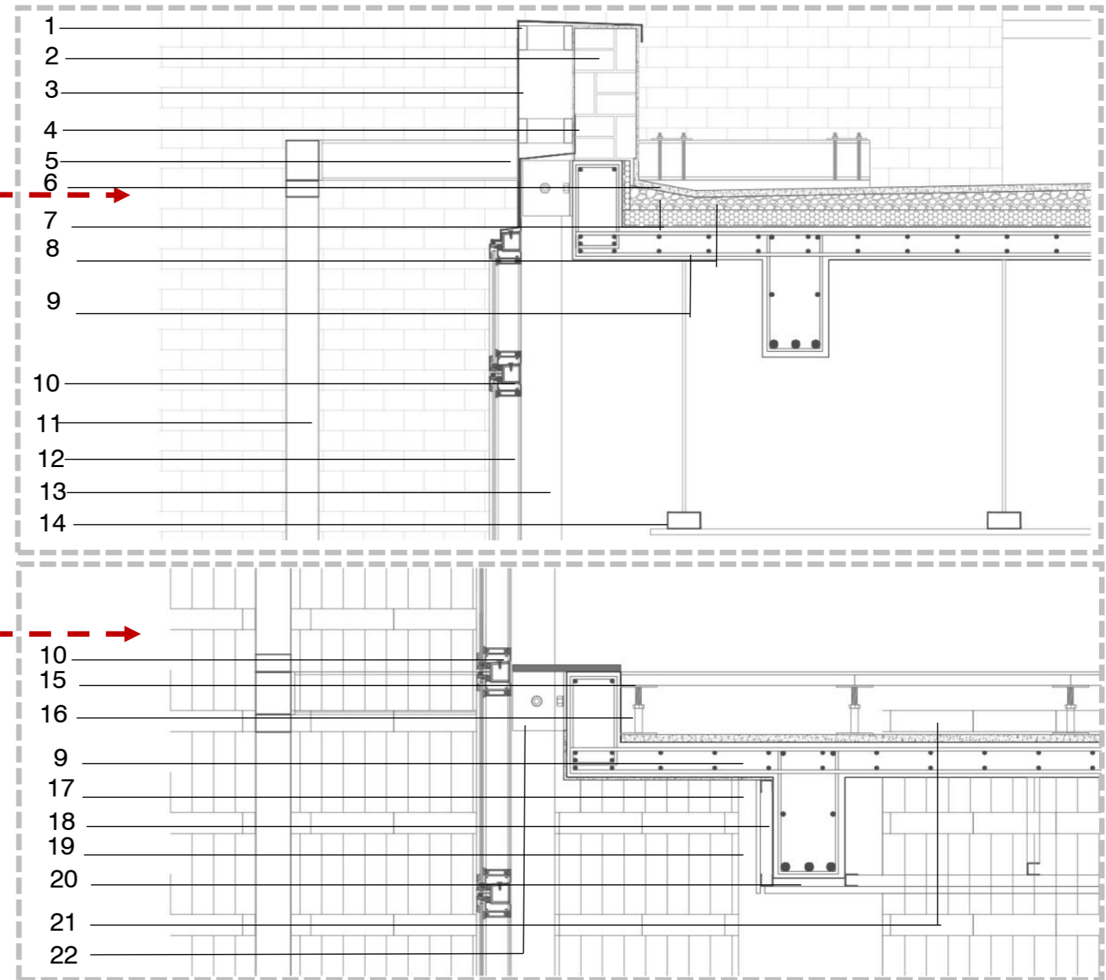
DETALLE 2: Entrepiso
