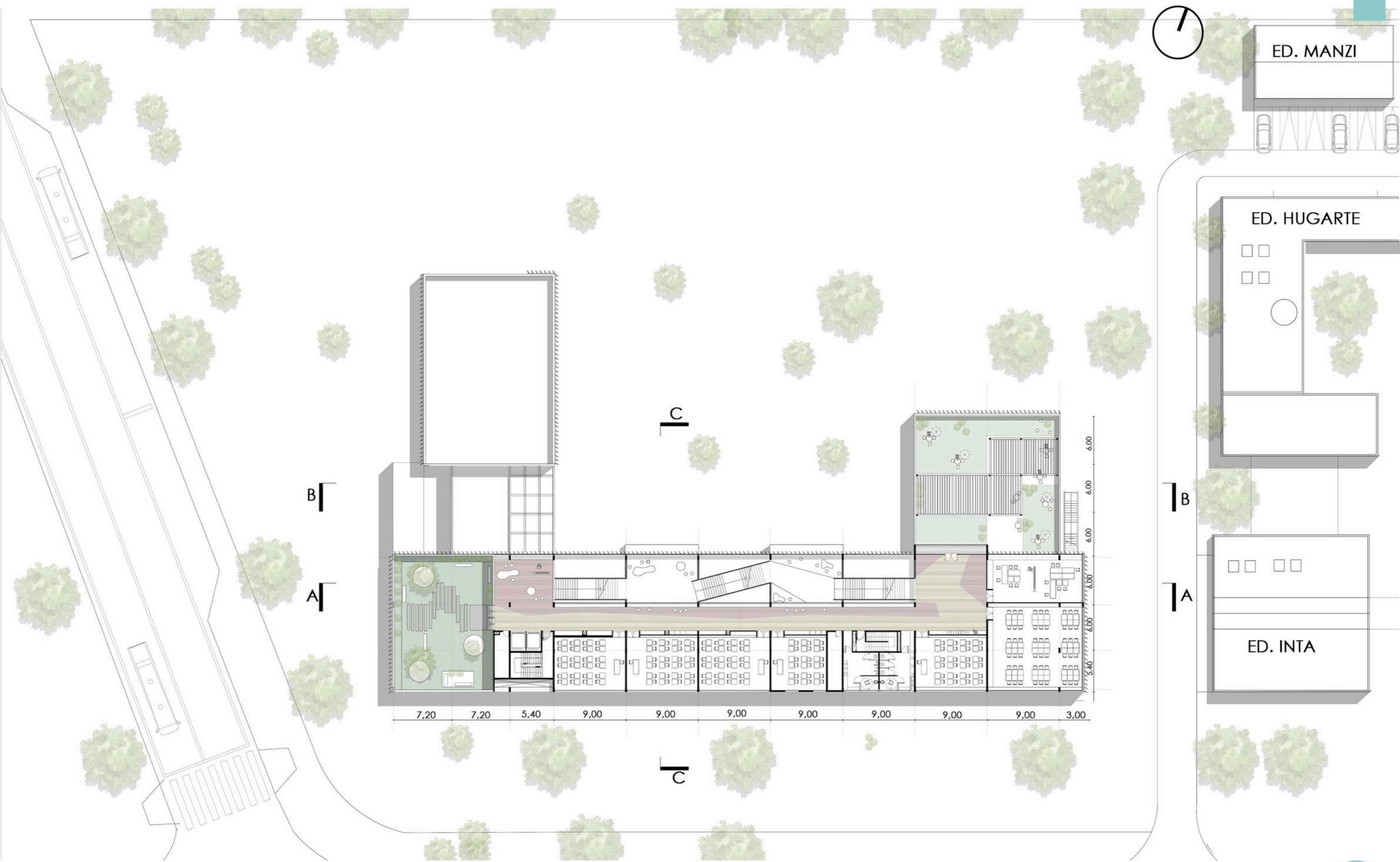
Planta tercera
