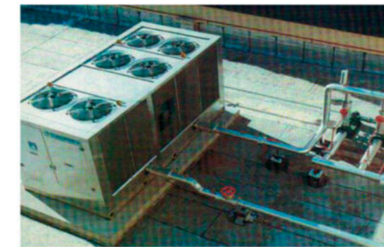
Máquina enfriadora de líquidos (MEL) condensada por aire, puede traer un kit hidráulico
