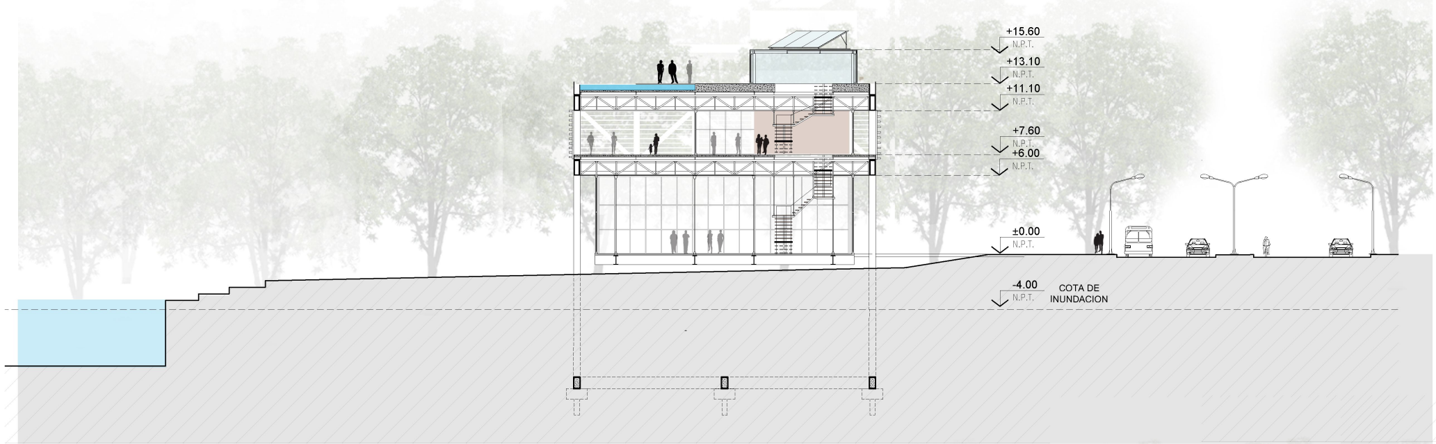
CORTE D-D
