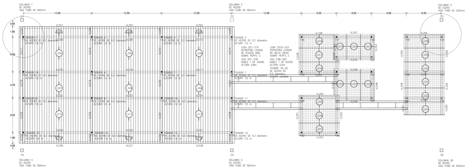
PLANTA ESTRUCTURA PLATAFORMAS
