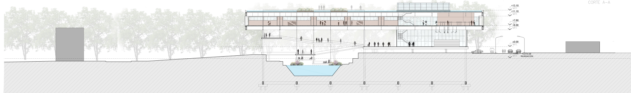
CORTE B-B
