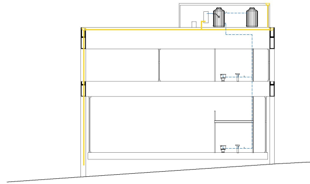
SISTEMA RECOLECCION DE AGUA DE LLUVIA ABASTECIMIENTO DE AGUA PARA USO SECUNDARIO (RIEGO - INODOROS - LIMPIEZA)
