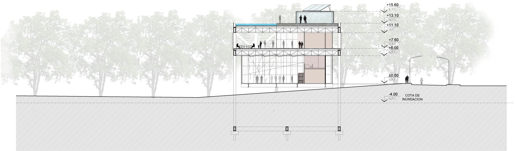
CORTE C-C
