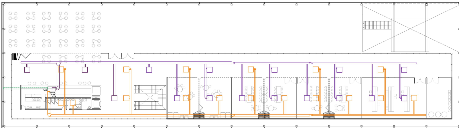
PLANTA ALTA
