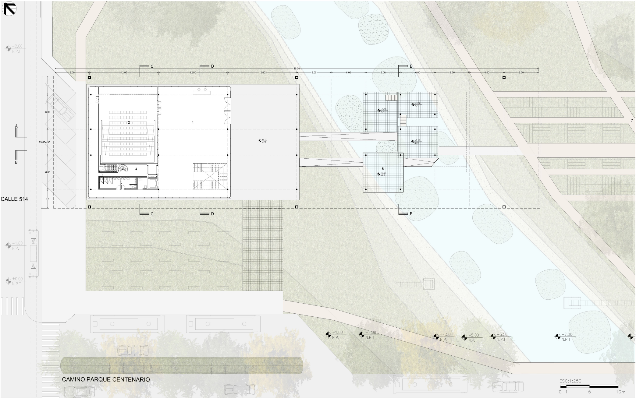
PLANTA BAJA
