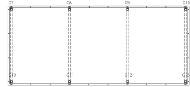
PLANTA ESTRUCTURA TERRAZA
