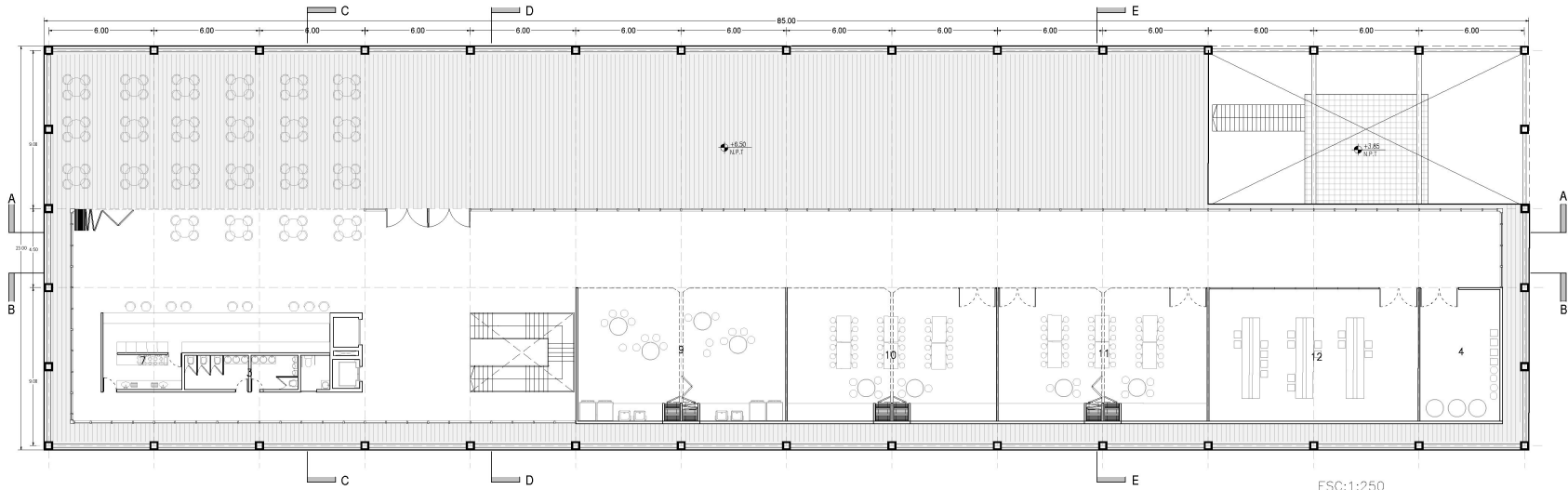
ESC:1:250 0 1 5 10m
